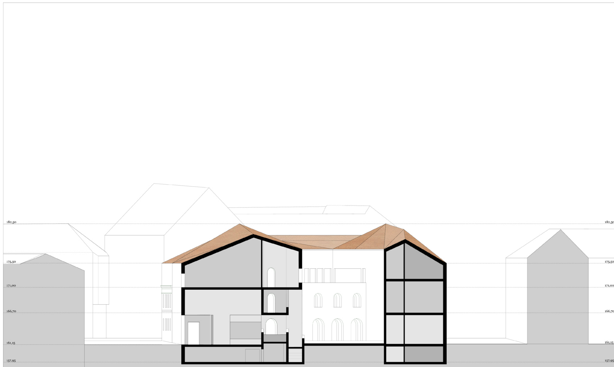
c - c metszet
