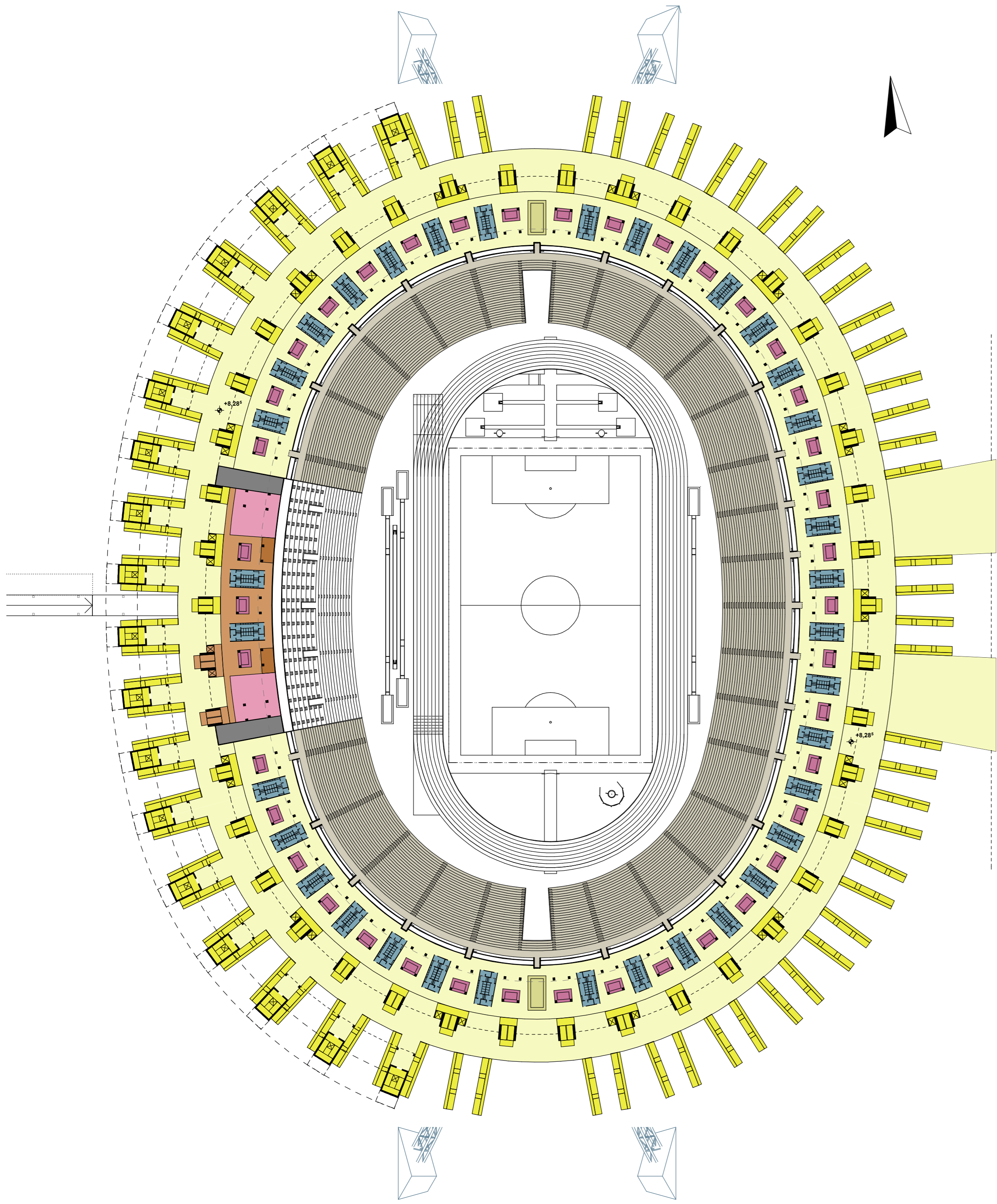
FŐSÉTÁNY SZINT ALAPRAJZ +8,28 M
