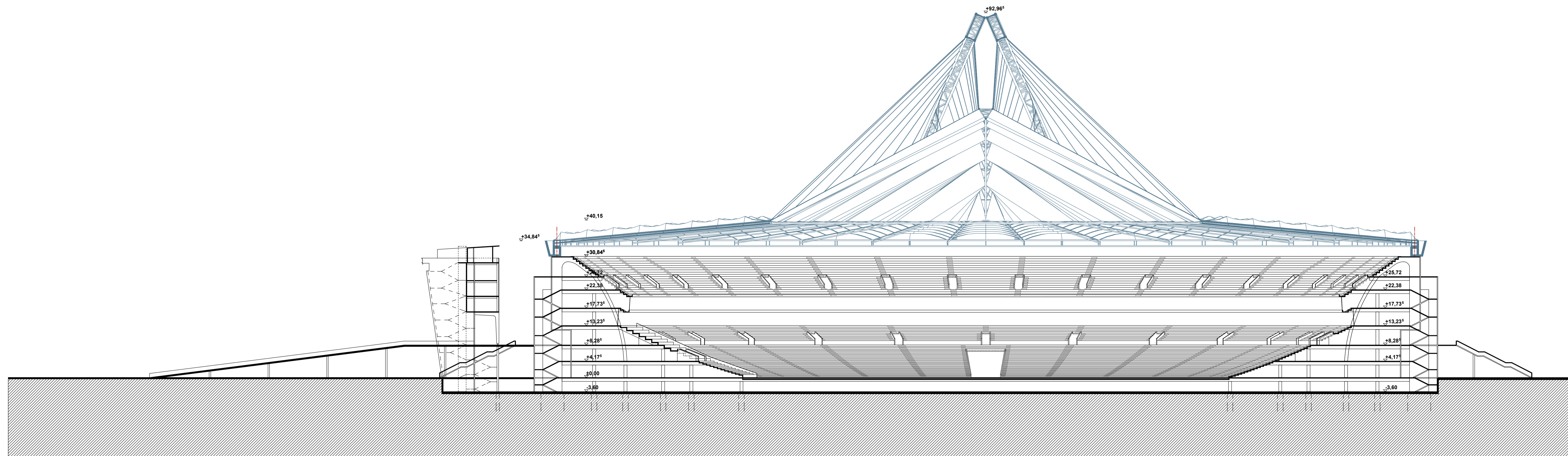
KERESZTMETSZET M=1:500
