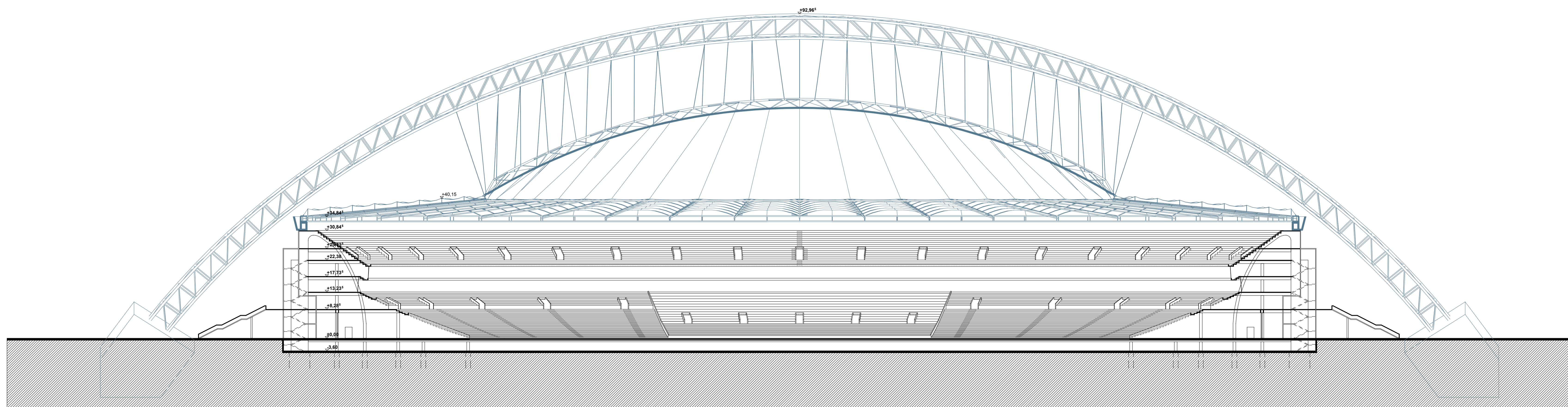
HOSSZMETSZET M=1:500
