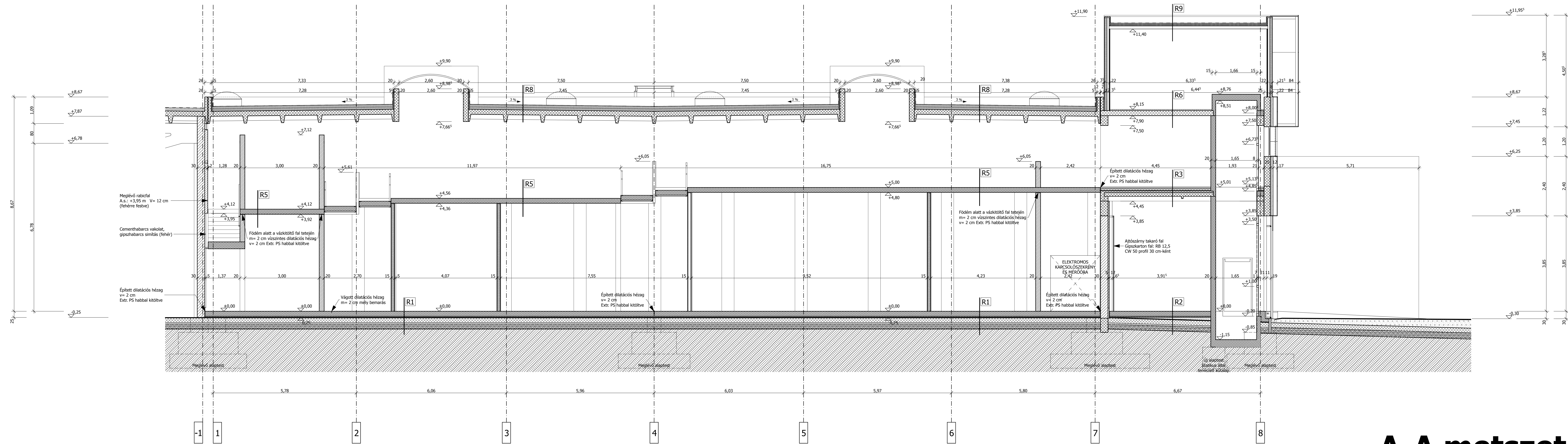
A-A metszet
