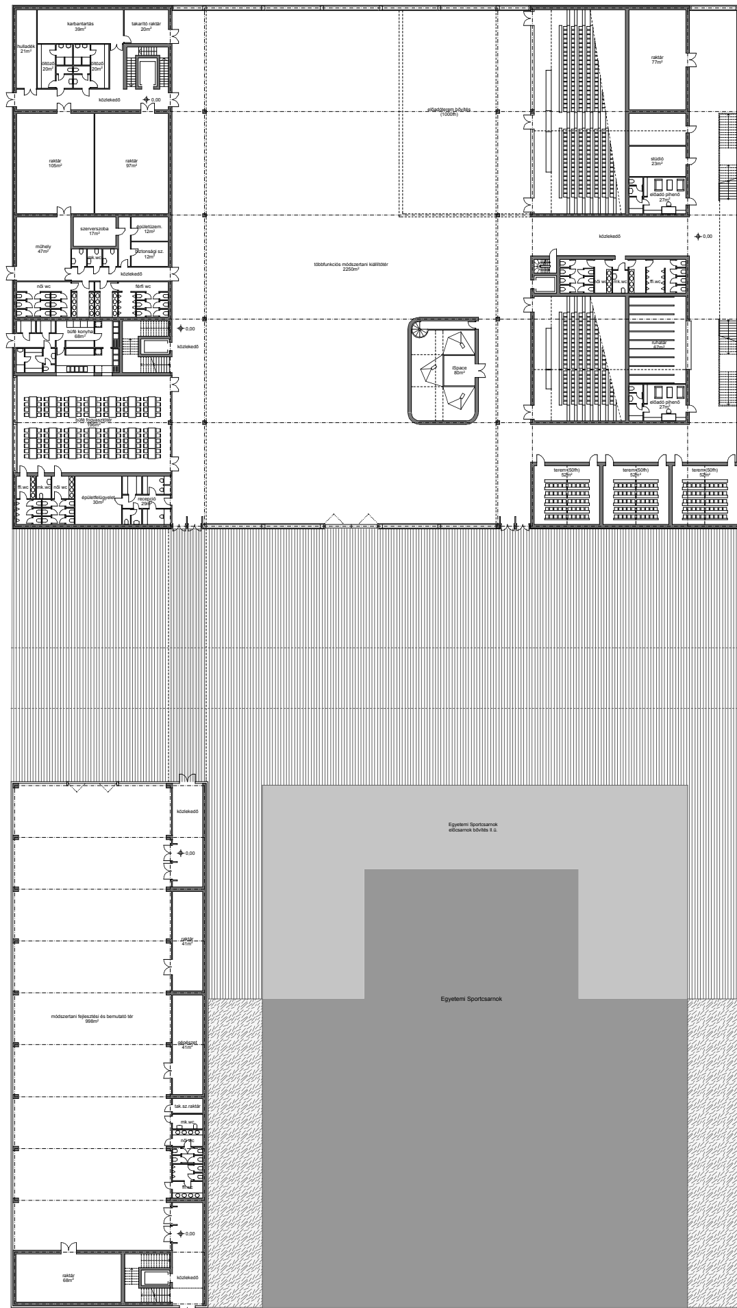
Movesmart alaprajz
