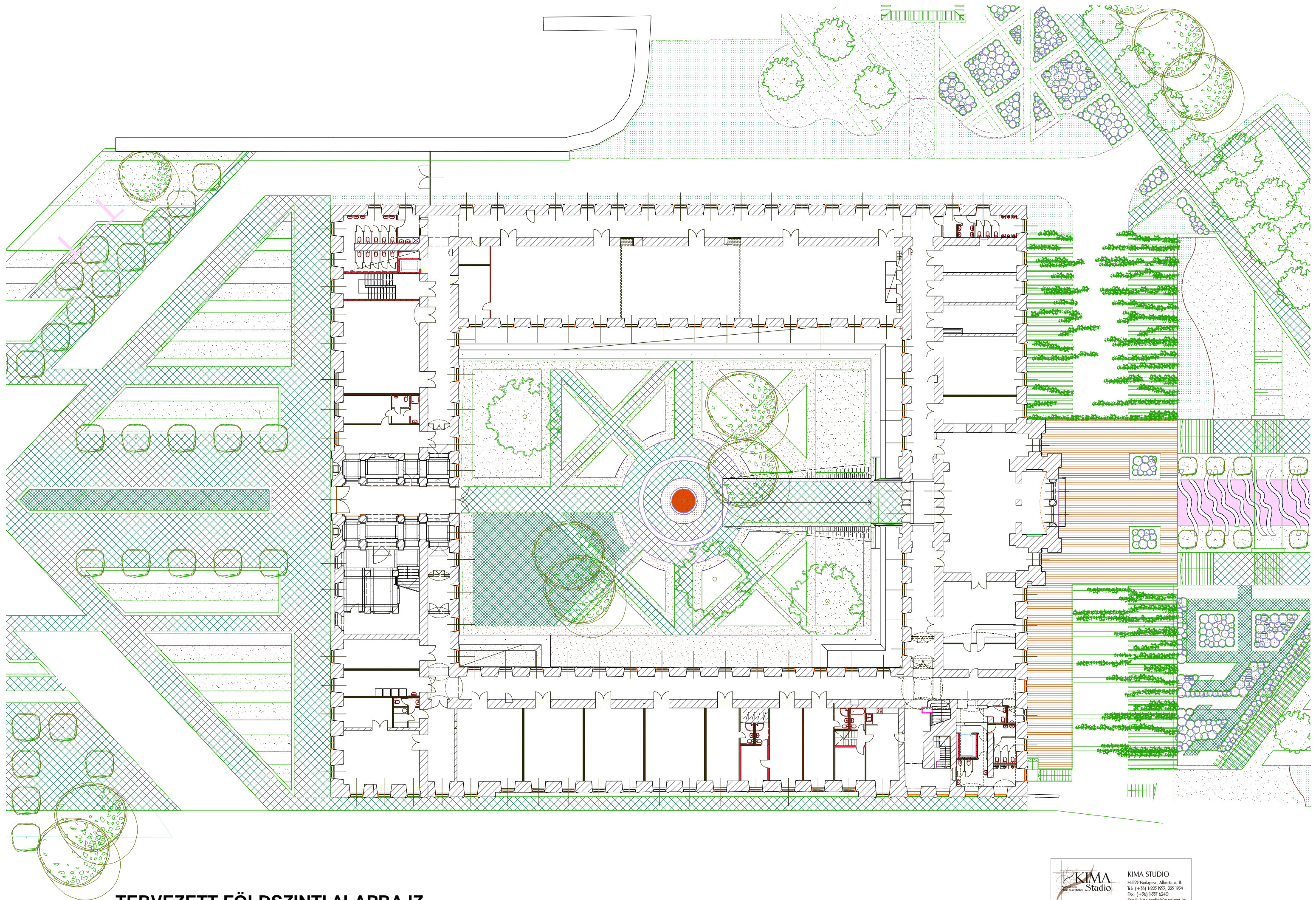
TERVEZETT FÖLDSZINTI ALAPRAJZ
