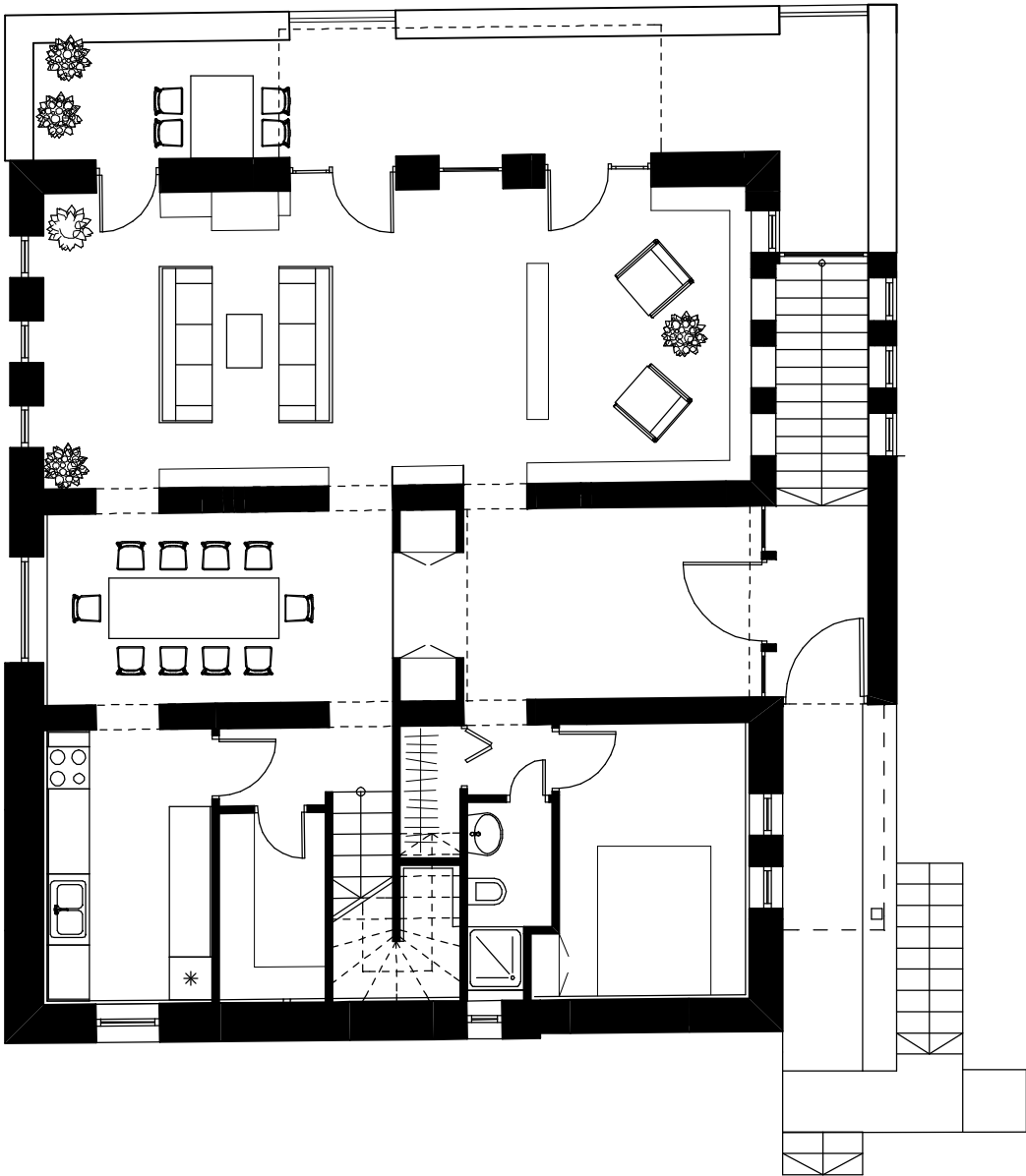
FÖLDSZINTI ALAPRAJZ M=1:100
