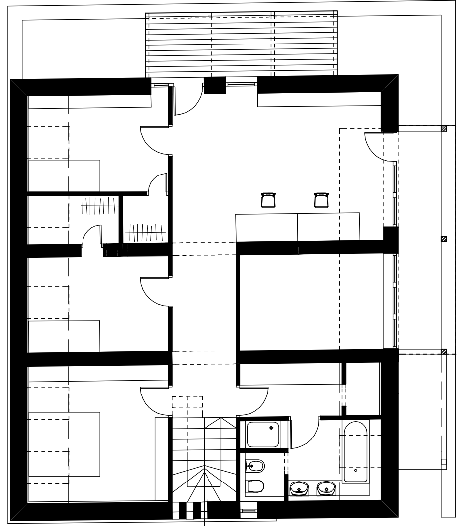
TETŐTÉRI ALAPRAJZ M=1:100
