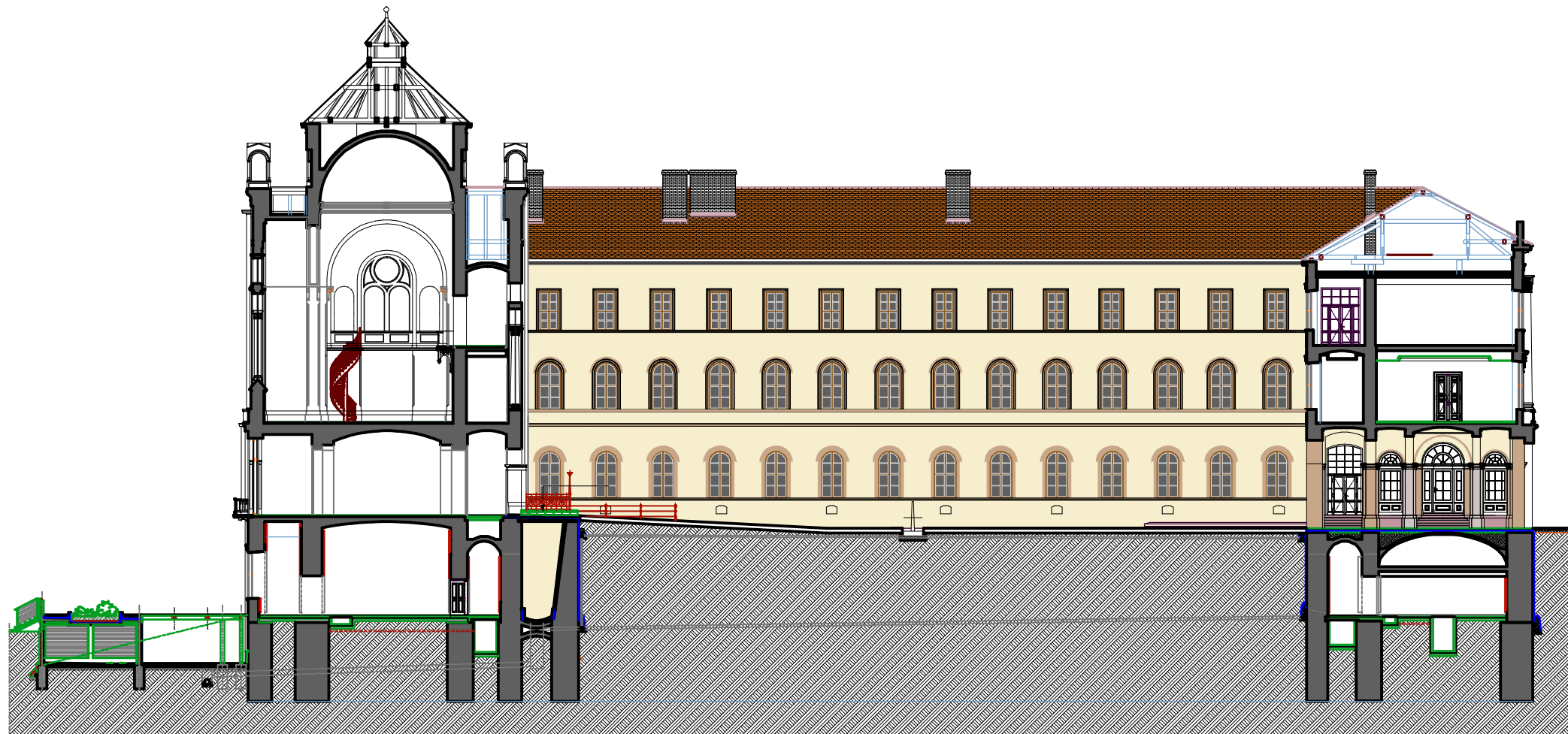
TERVEZETT C-C METSZET
