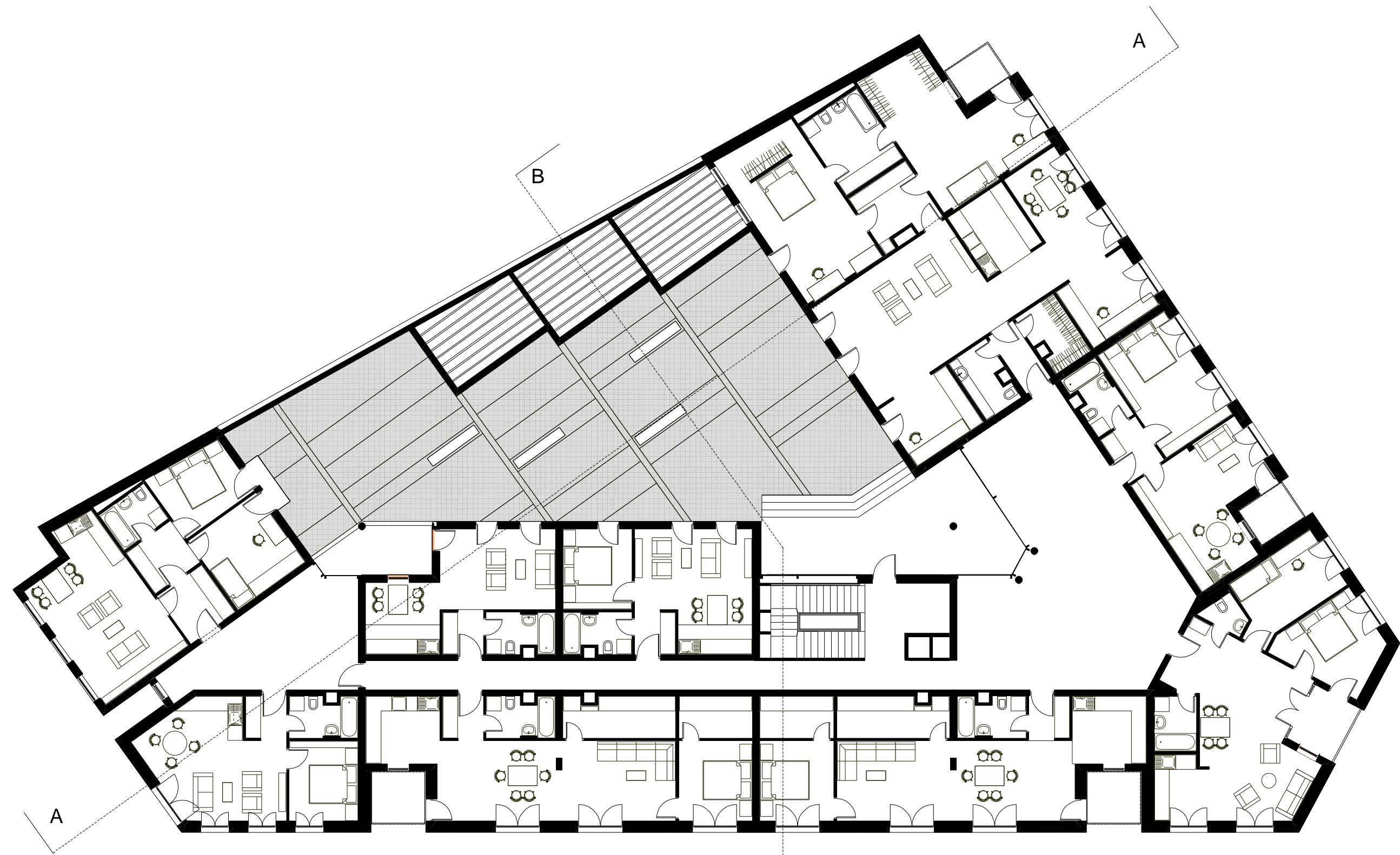
Újpest városközpont . Kemény Gusztáv utcai 35 lakásos társasház, 1.emeleti alaprajz
