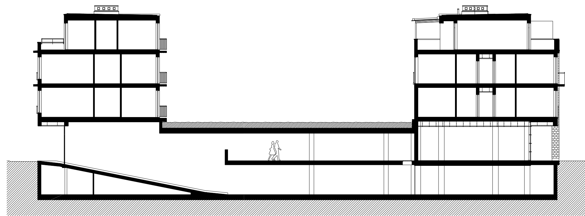
Újpest városközpont . Kemény Gusztáv utcai 35 lakásos társasház, A-A metszet
