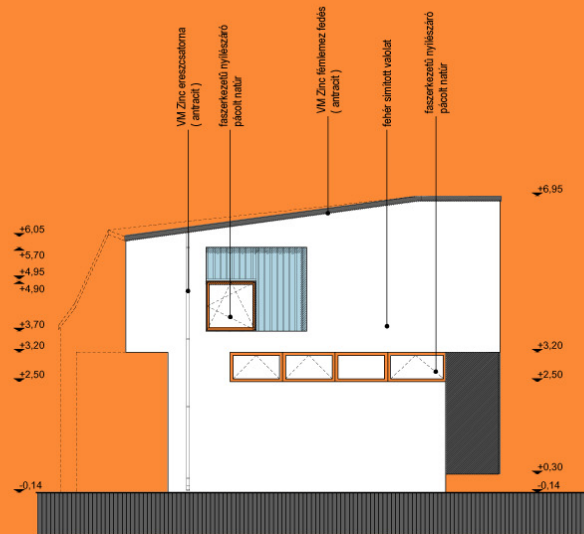
DÉL-NYUGATI HOMLOKZAT
