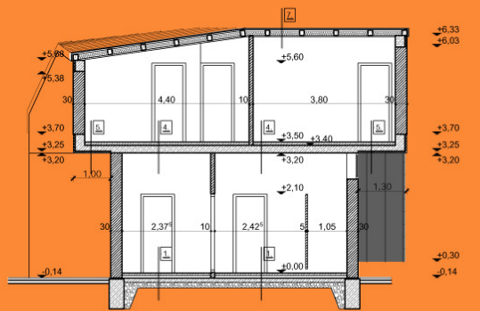
E - E METSZET
