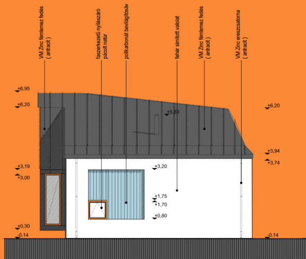
ÉSZAK-KELETI HOMLOKZAT
