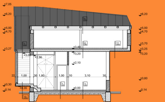
D - D METSZET
