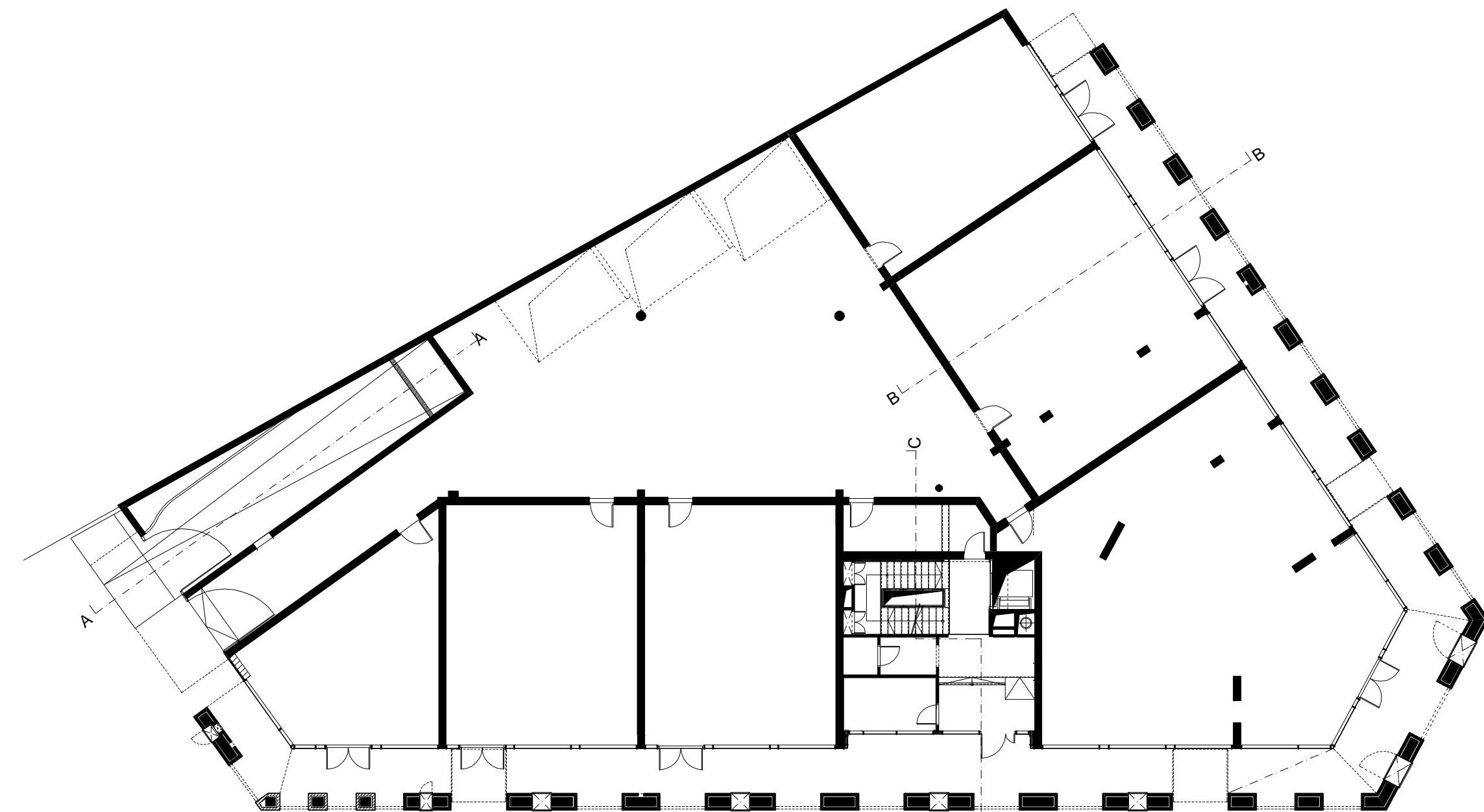
Újpest városközpont . Kemény Gusztáv utcai 35 lakásos társasház, földszinti alaprajza
