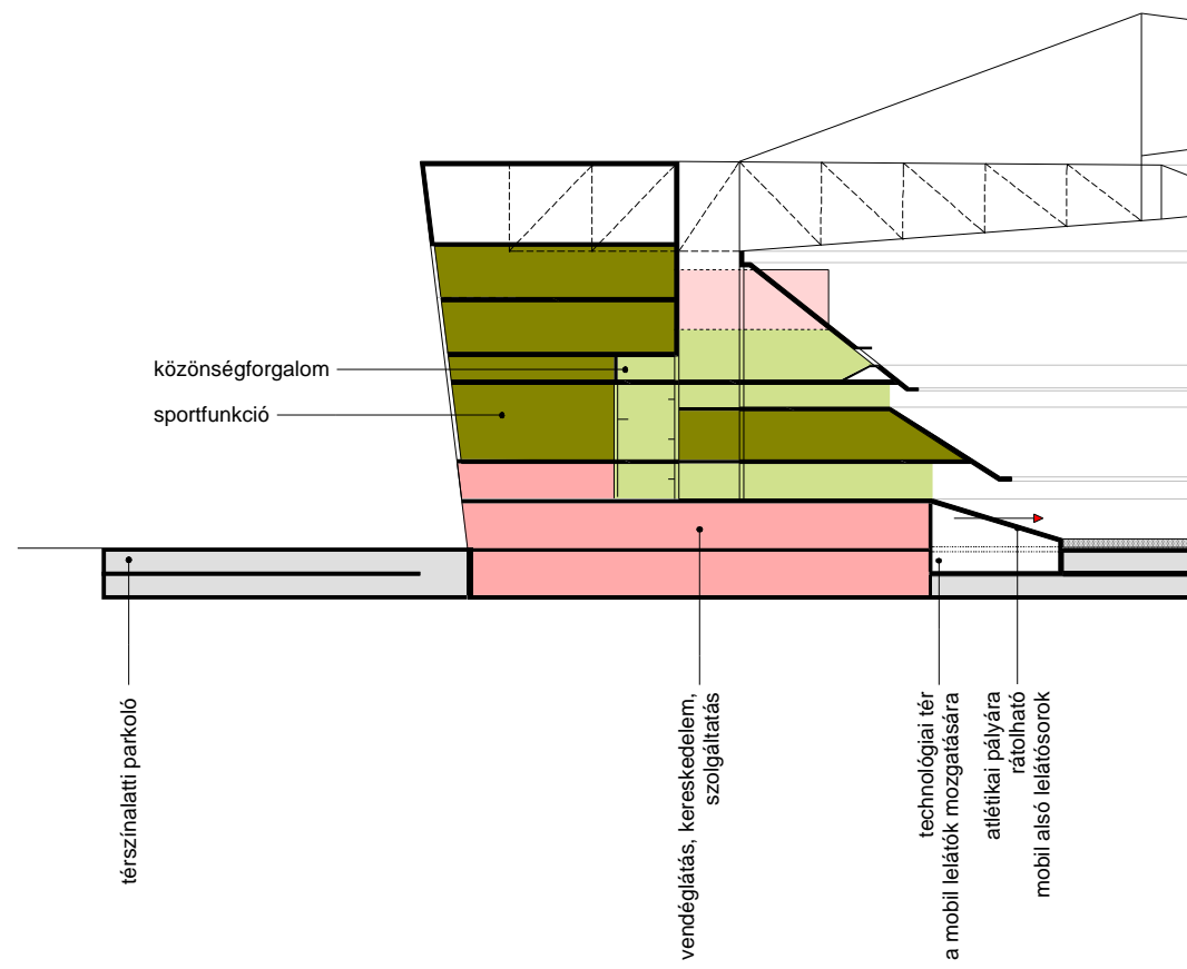
B-B METSZET M 1:2000
