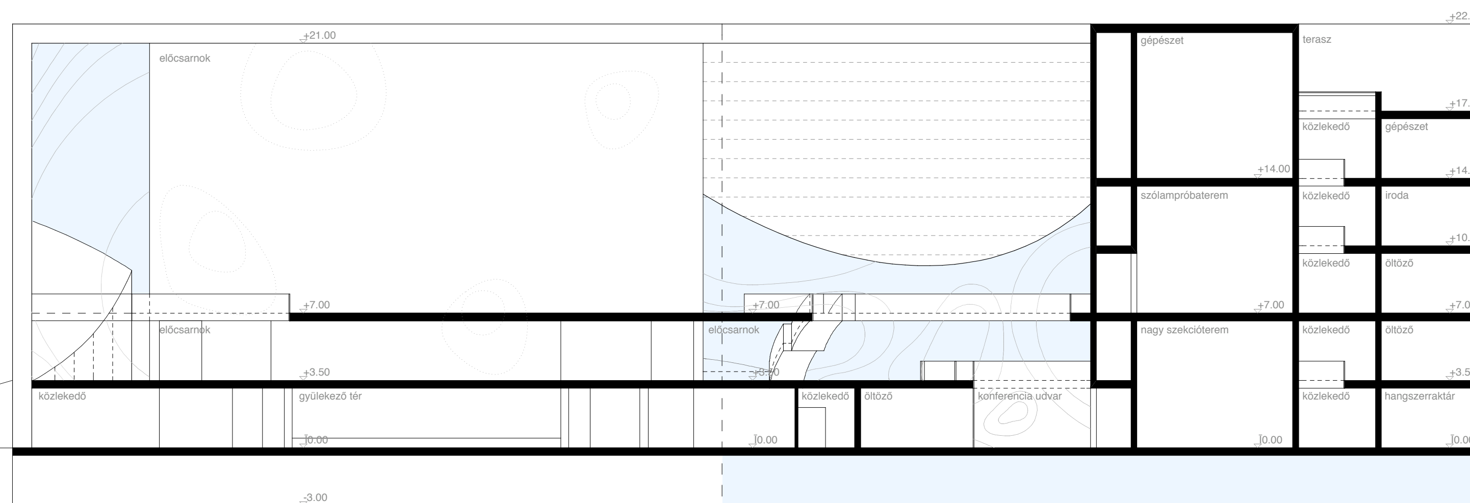
3_3 metszet m 1:200
