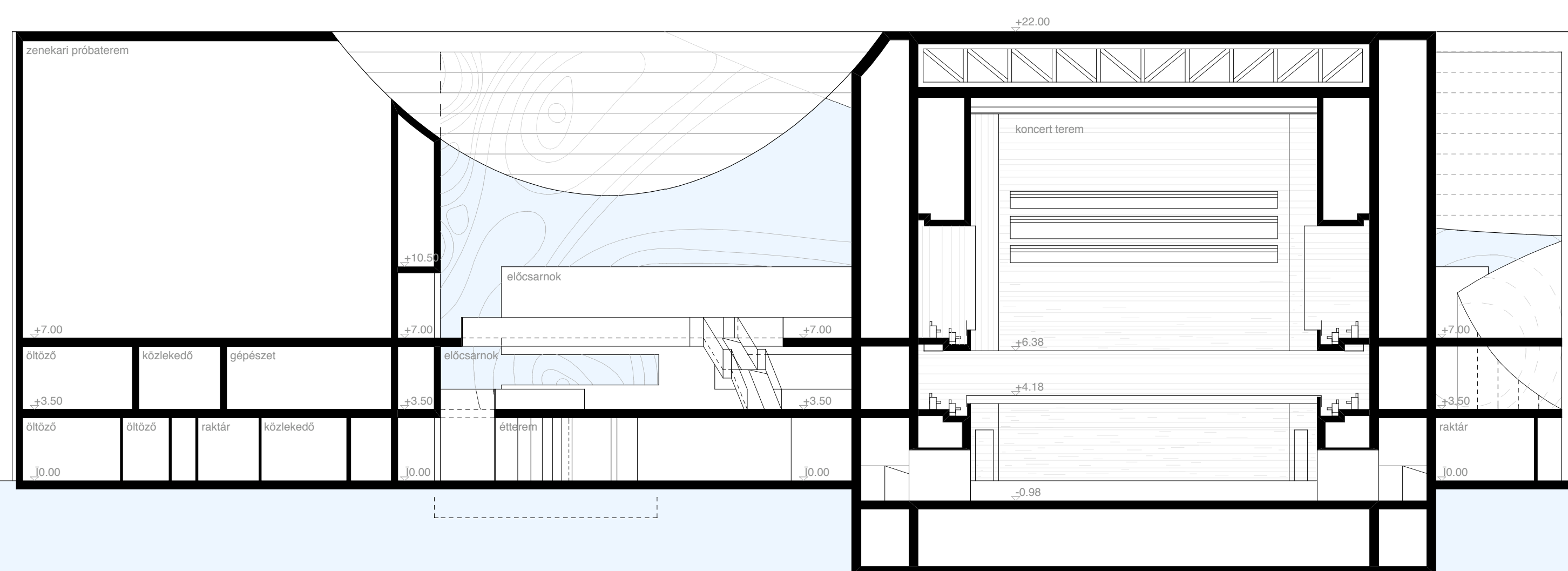
2_2 metszet m 1:200
