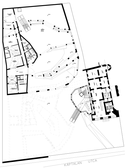
NAGY KIÁLLÍTÓTÉR - 1. EMELÉTI ALAPRAJZ, KÖZÖSSÉGI FŐL 1/100
