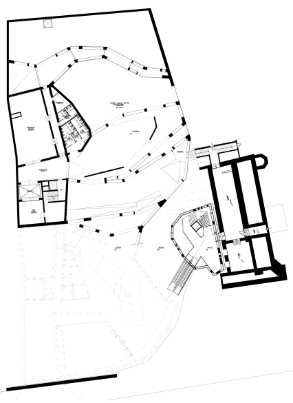
NAGY KIÁLLÍTÓTÉR - 2. EMELÉTI ALAPRAJZ, NAGY KIÁLLÍTÓTÉR, 1/100
