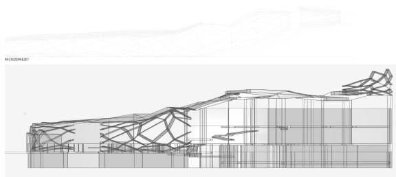
HOSSZMETSZET 1/100
