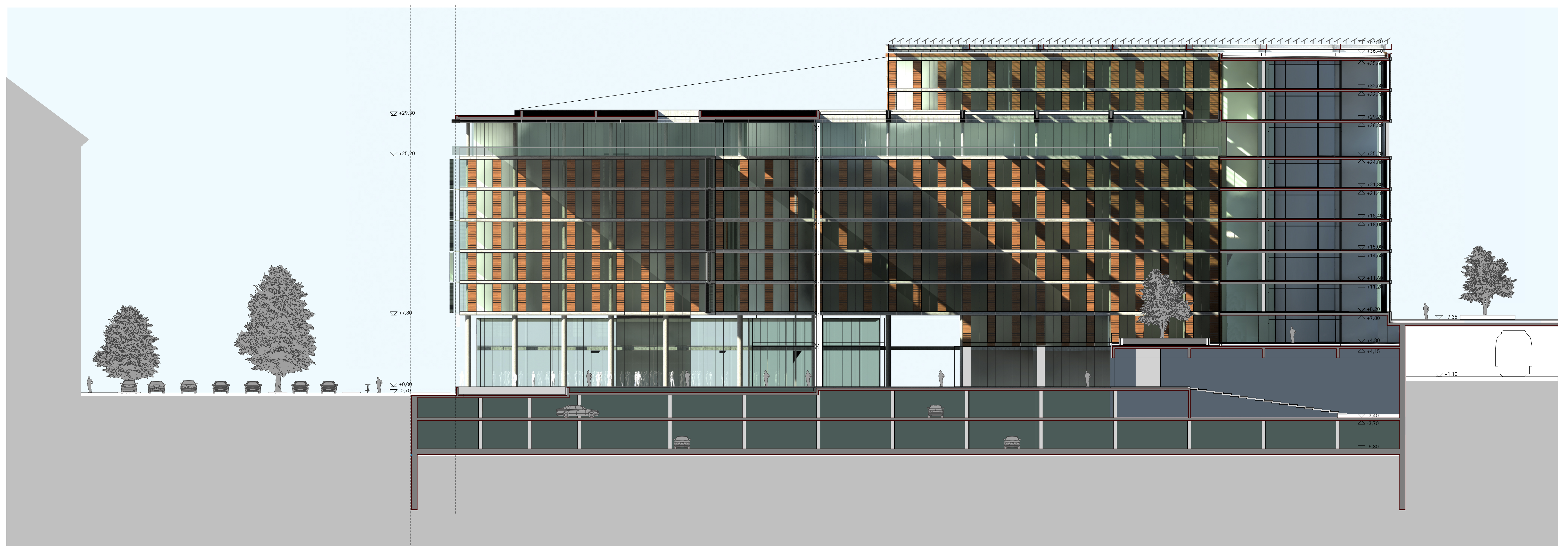
A-A METSZET
