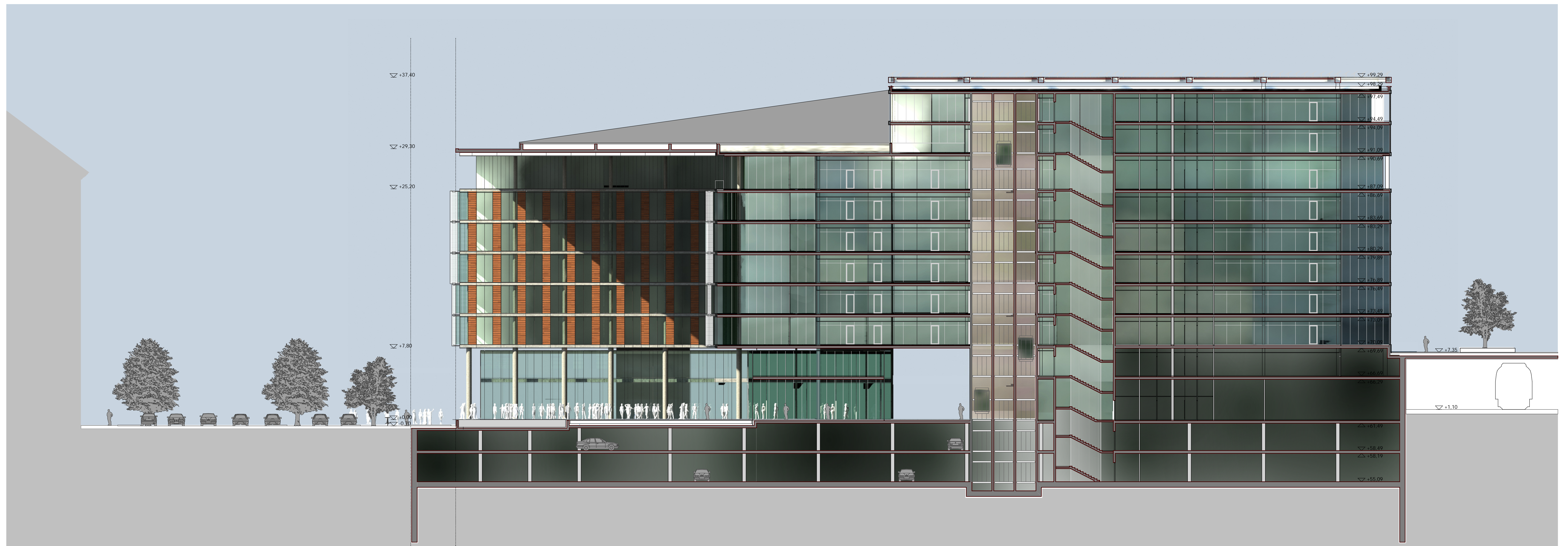
B-B METSZET
