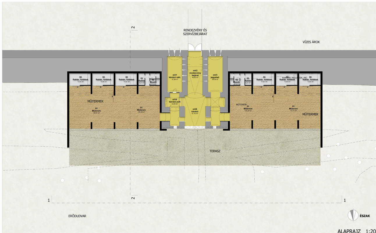
ALAPRAJZ 1:200
