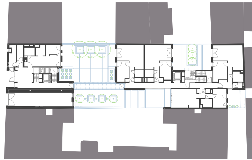
02 FÖLDSZINT 1/m
