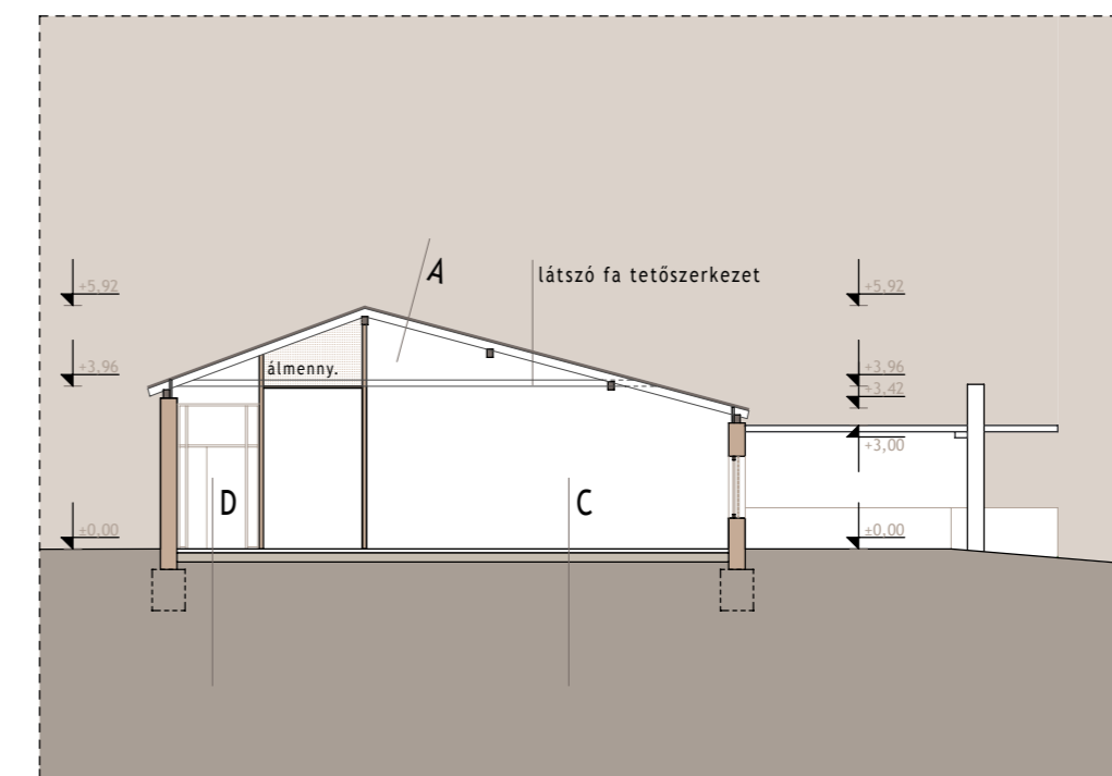
C - C metszet
