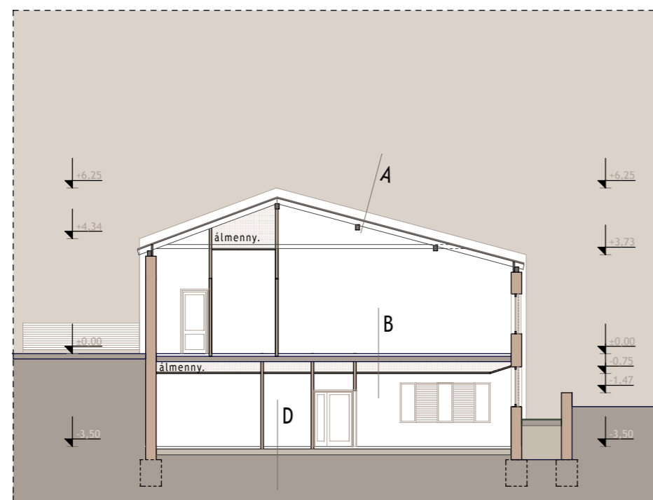
A - A metszet
