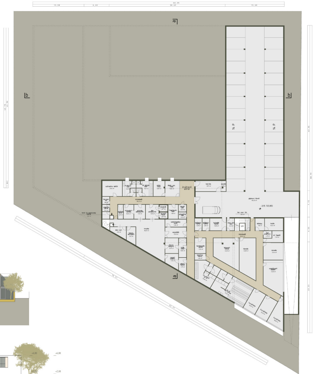
pincszinti alaprajz
