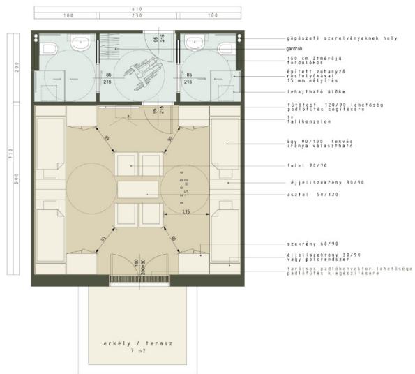
négyágyas szoba m=1:50
