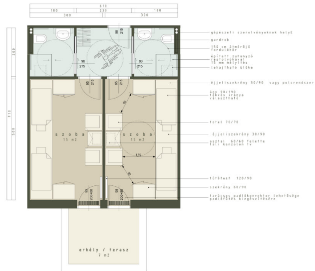
kétágyas szoba m=1:50
