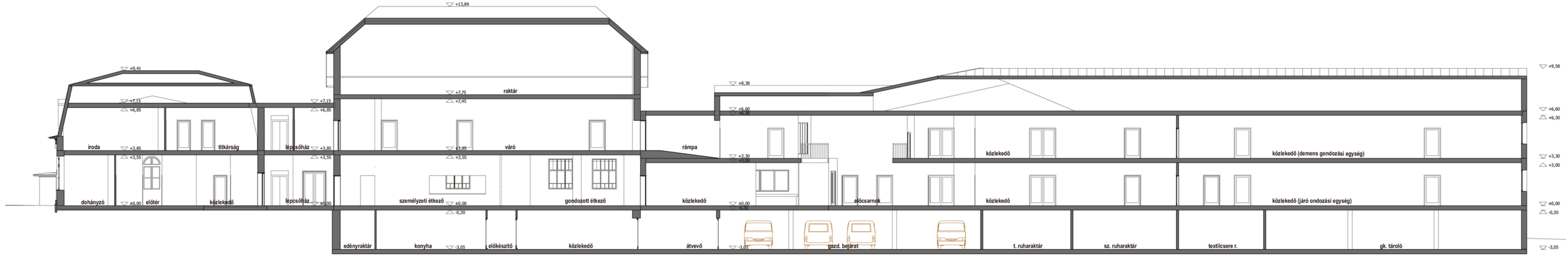
B-B metszet
