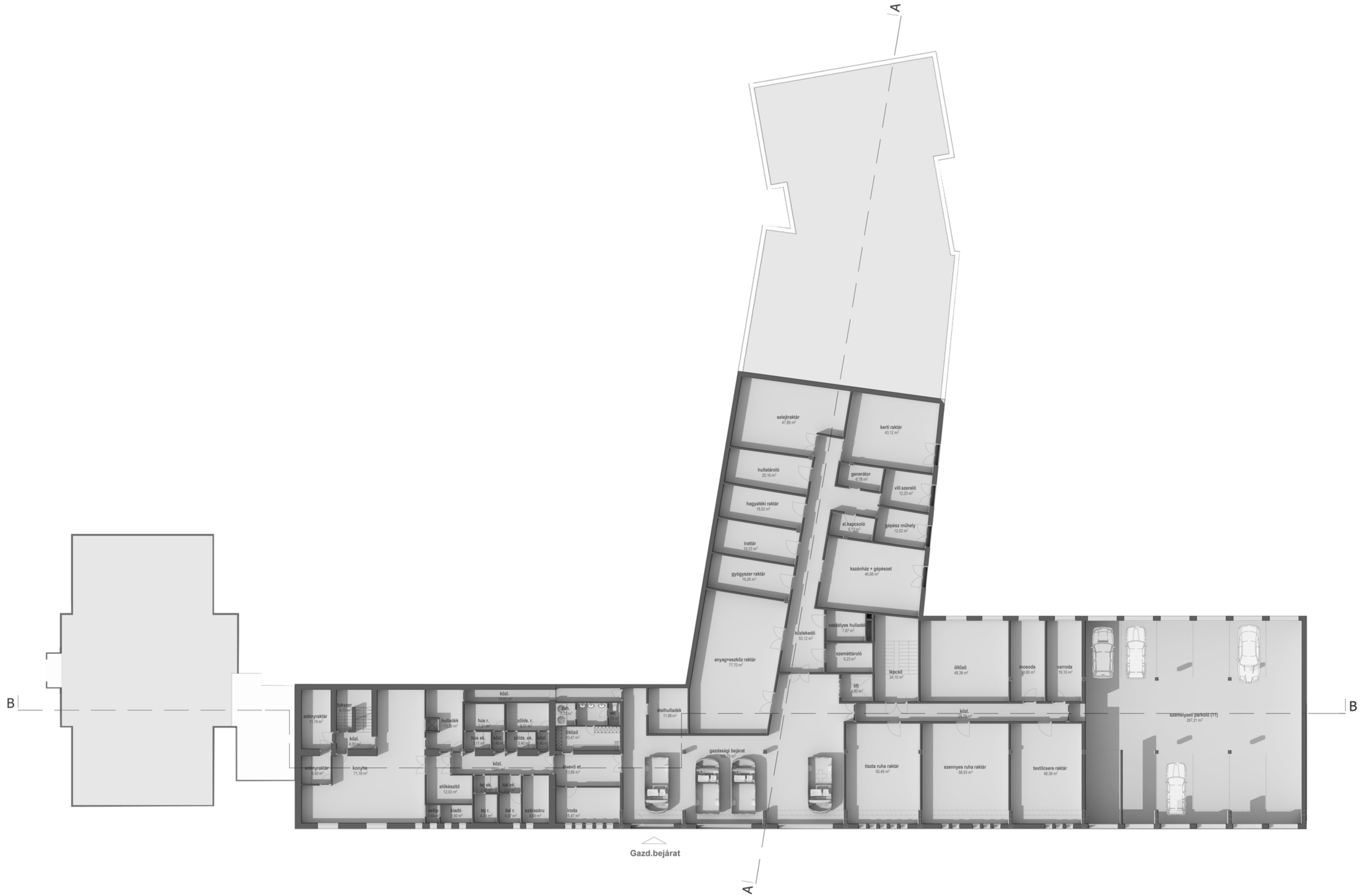
pince alaprajz
