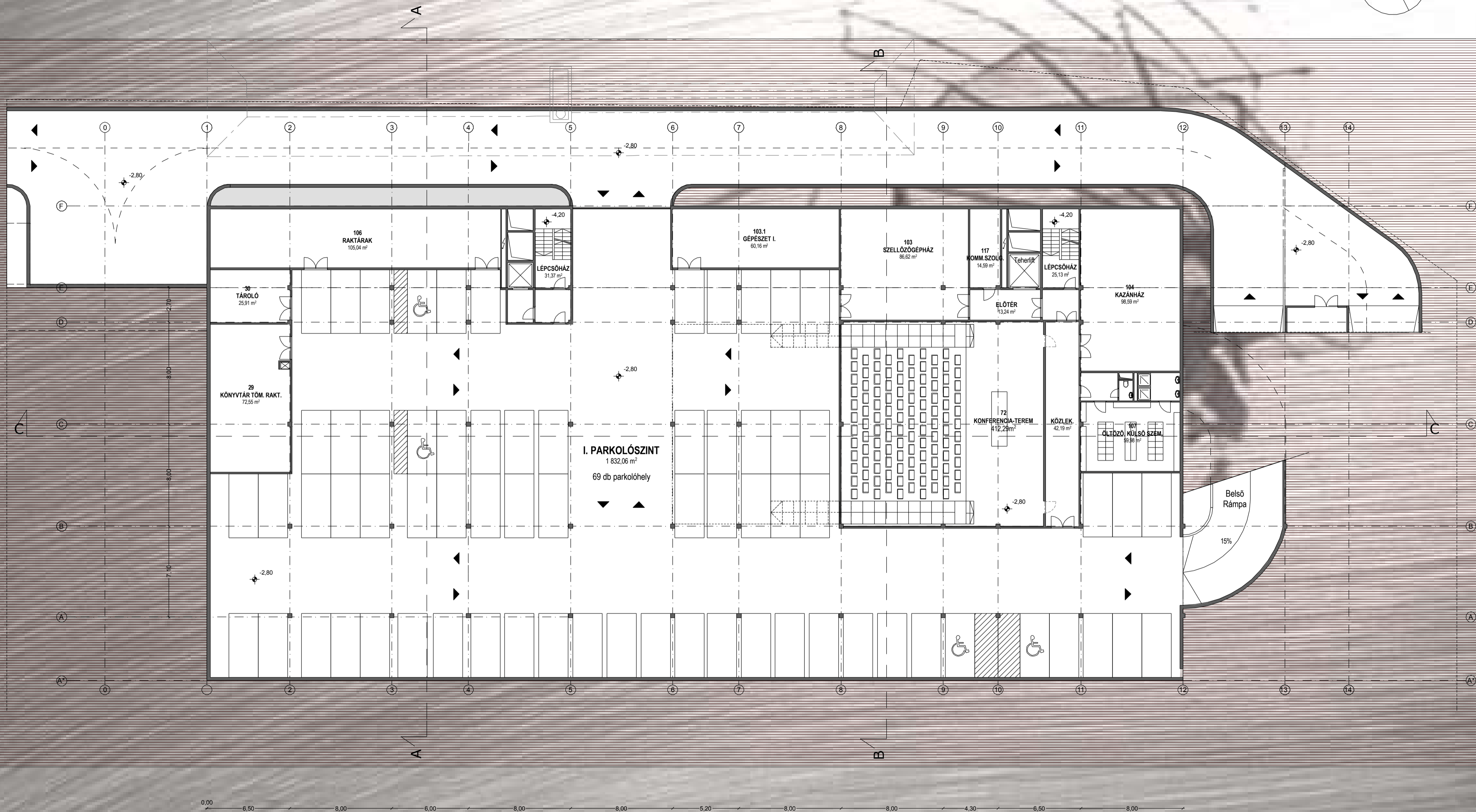
-1 PINCESZINT ALAPRAJZ M 1:200
