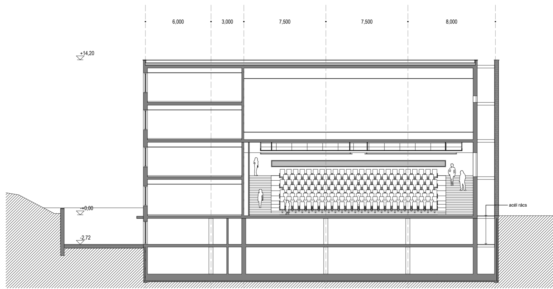
D-D METSZET
