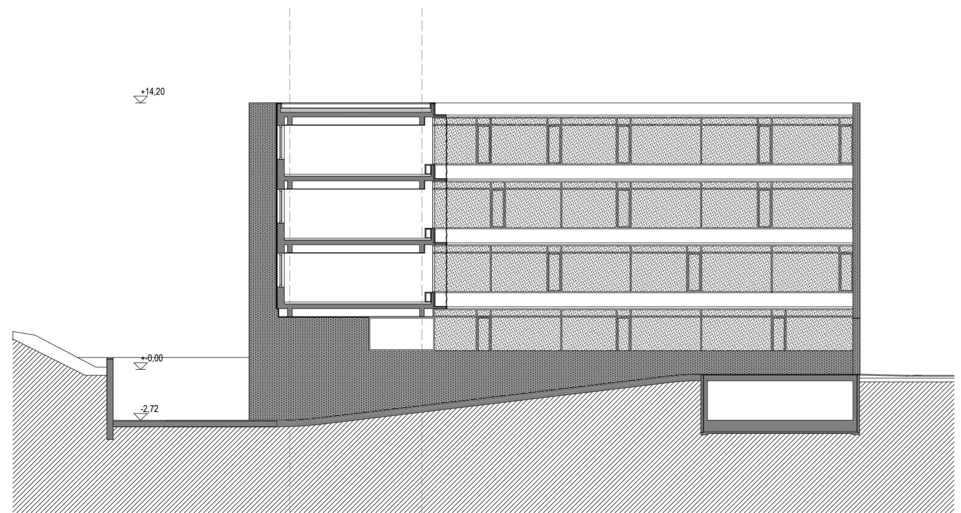
B - B METSZET
