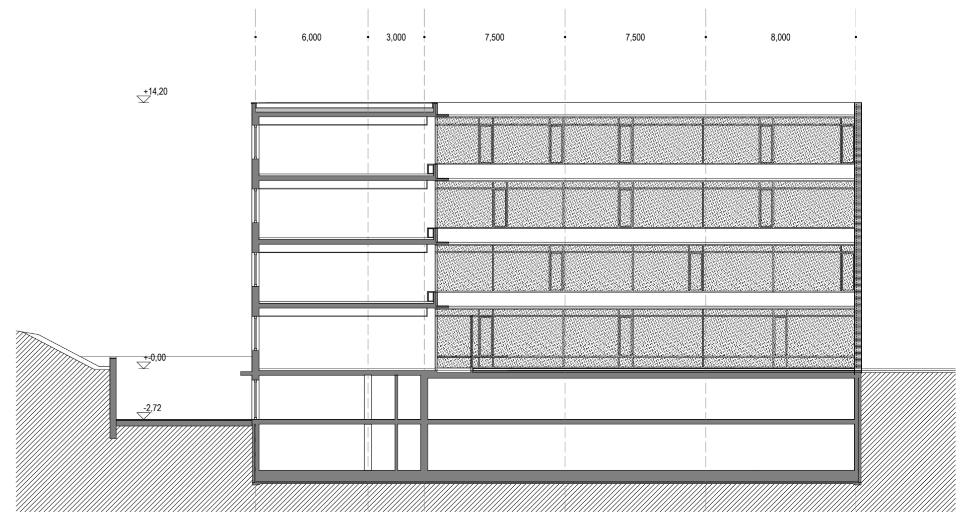
C - C METSZET
