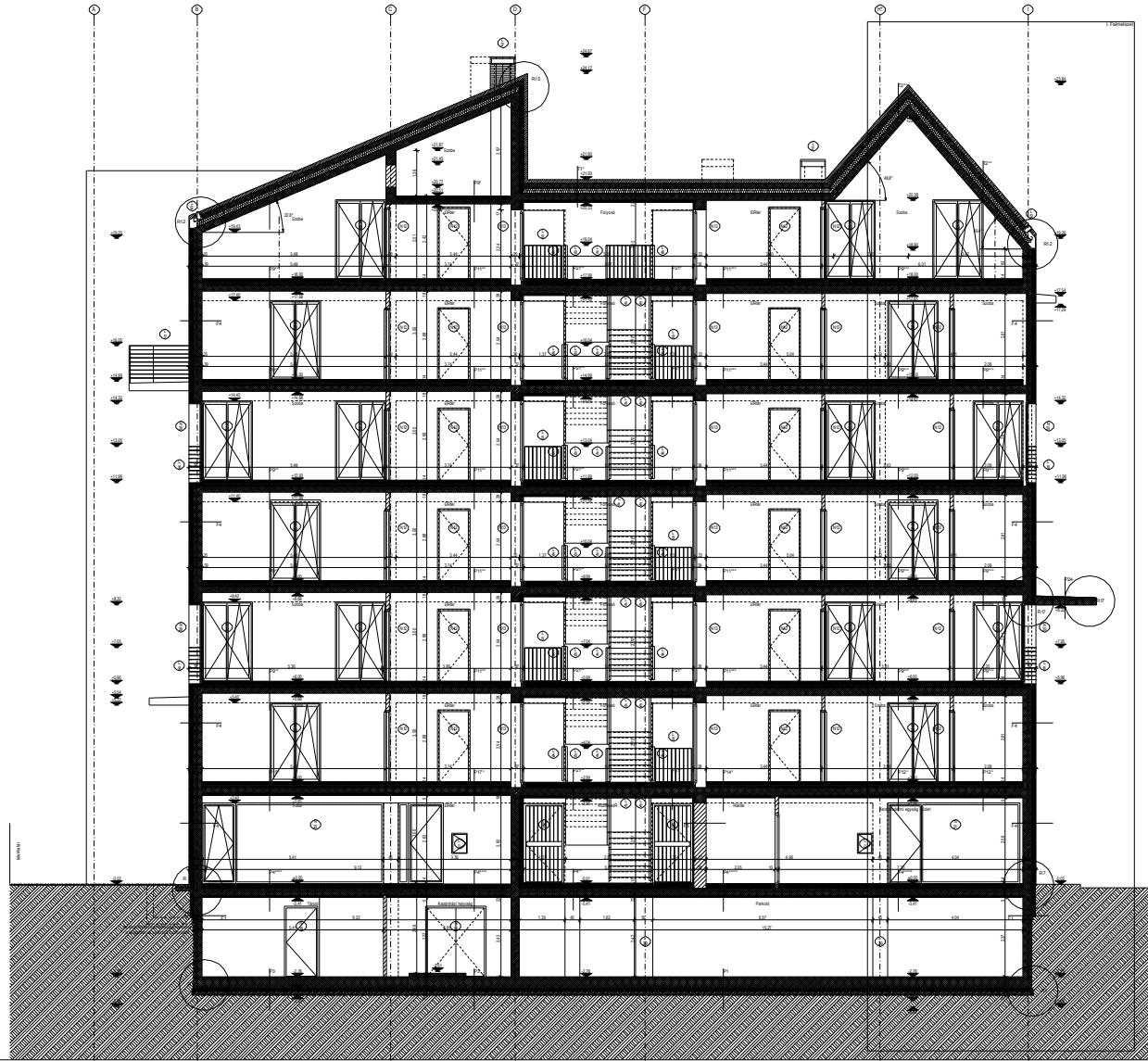
D-D metszet
