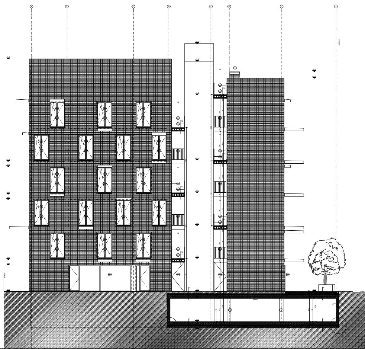
H-H metszet
