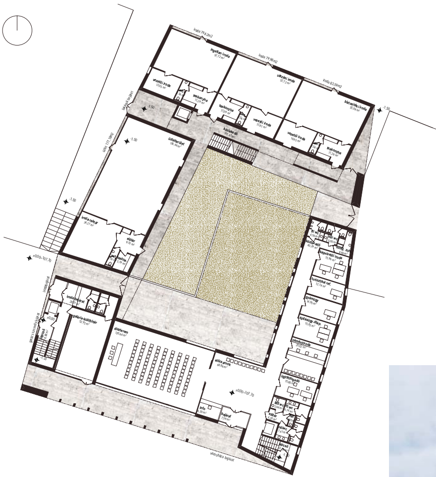
FÖLDSZINTI ALAPRAJZ M 1:200
