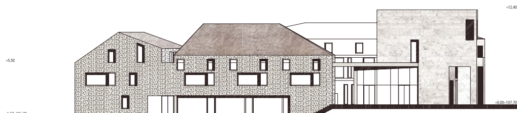
NYUGATI HOMLOKZAT M 1:200
