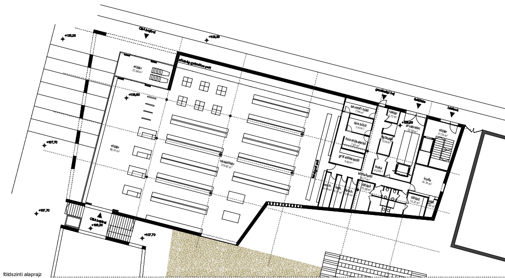
földszinti alaprajz
