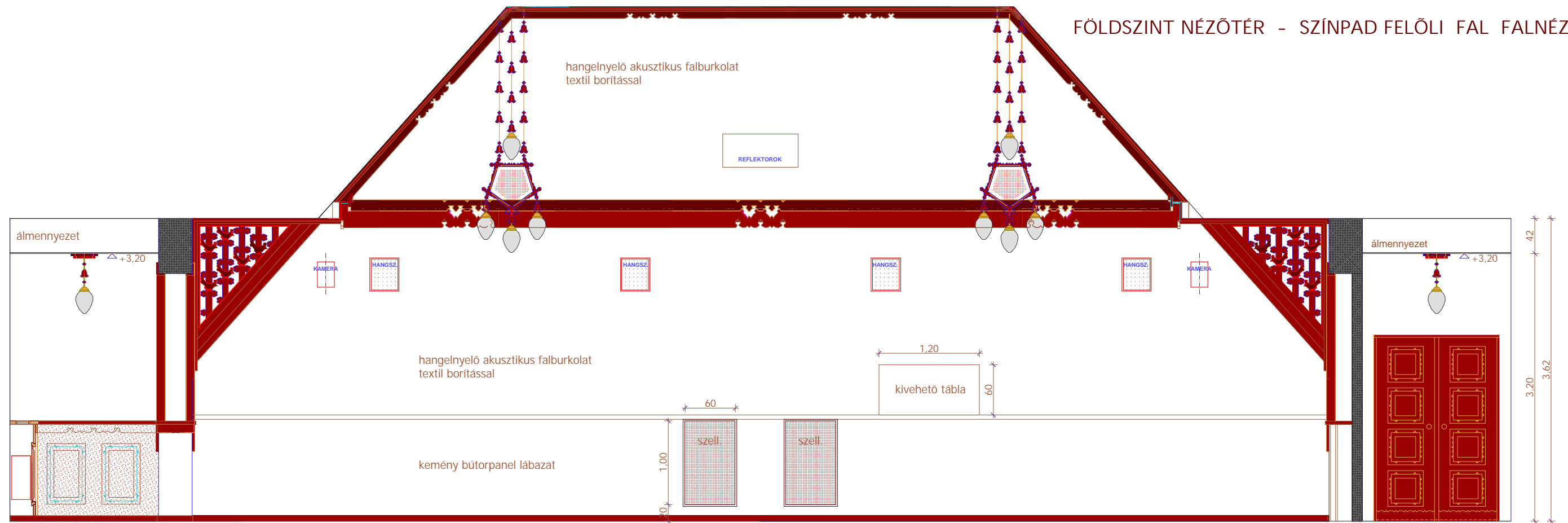
FÖLDSZINT NÉZŐTÉR - HÁTSÓ FAL FALNÉZETE
