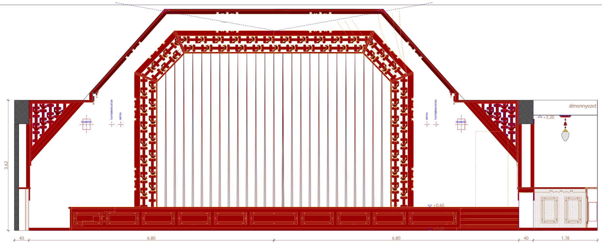
FÖLDSZINT NÉZŐTÉR - SZÍNPAD FELŐLI FAL FALNÉZETE
