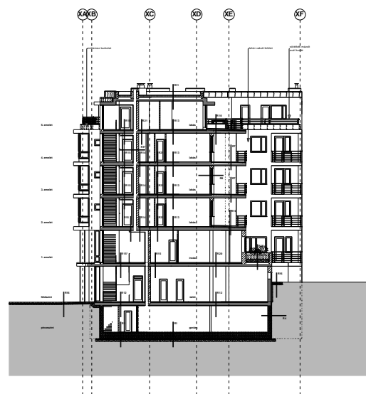
c-c metszet
