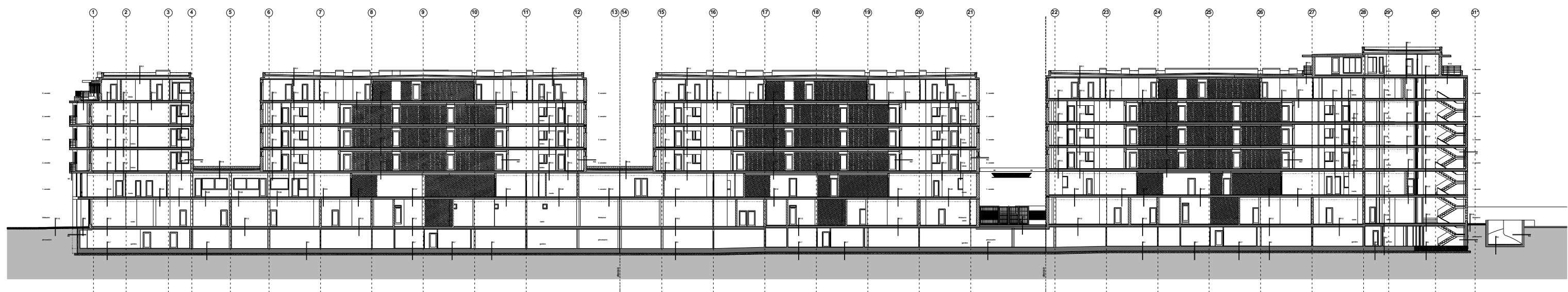
a-a metszet
