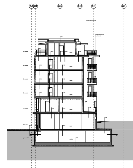
d-d metszet
