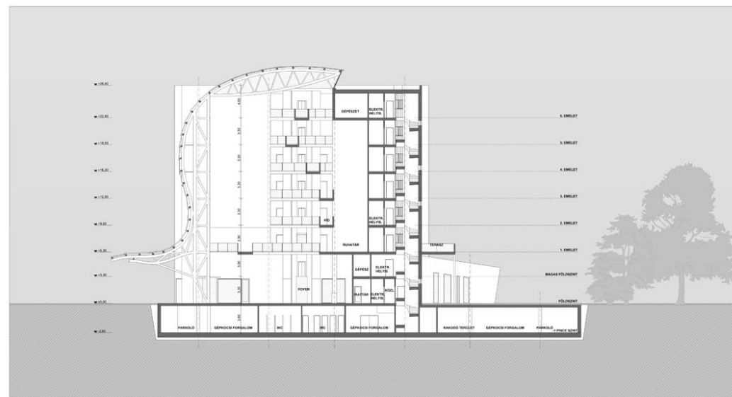
2-2 METSZET M 1:200
