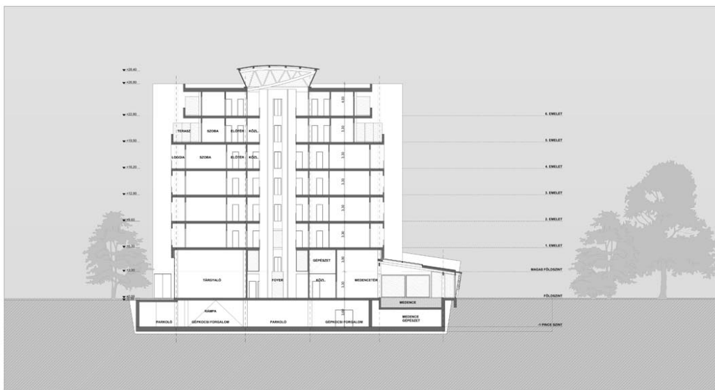
1-1 METSZET M 1:200
