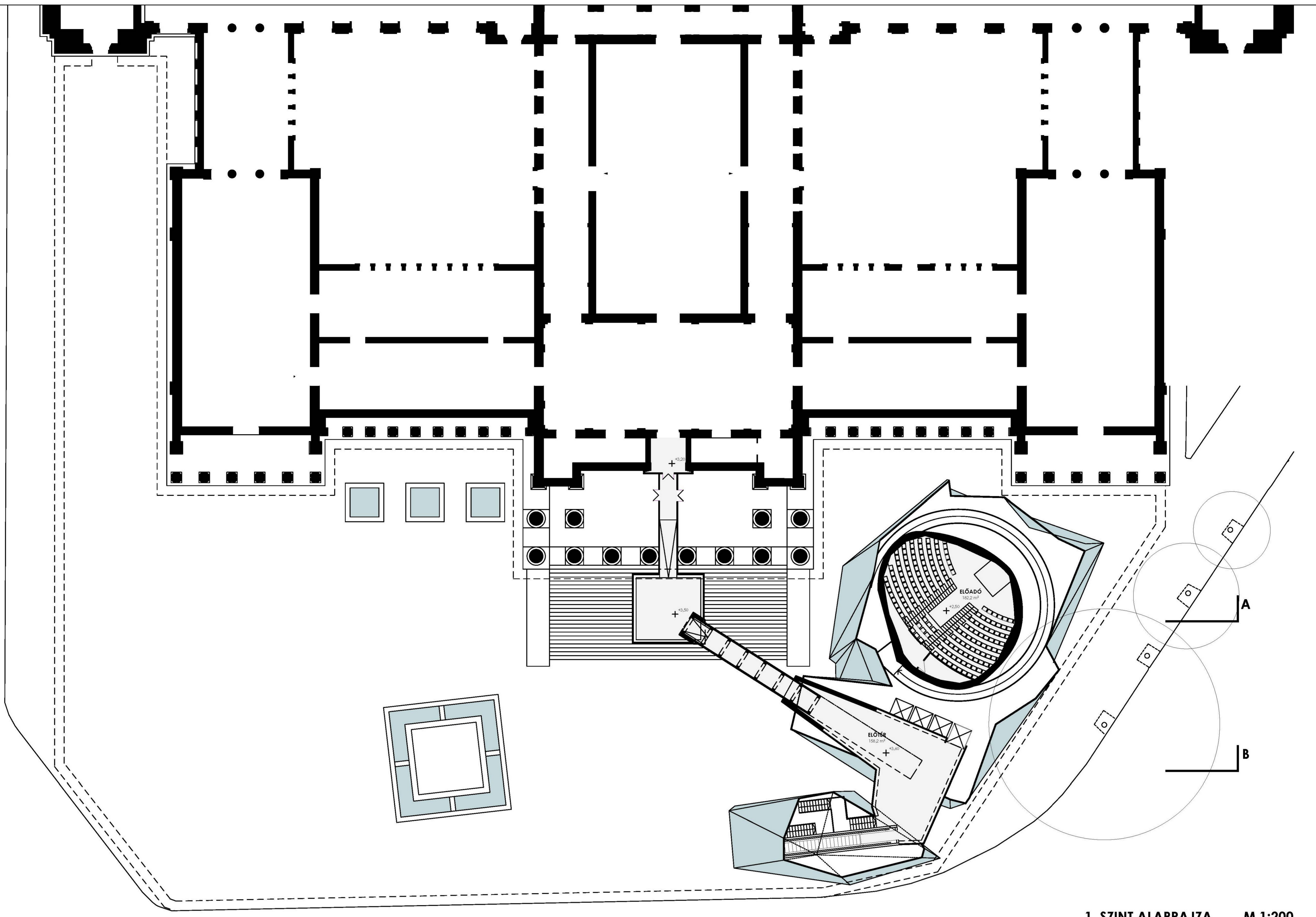
1. SZINT ALAPRAJZA M 1:200
