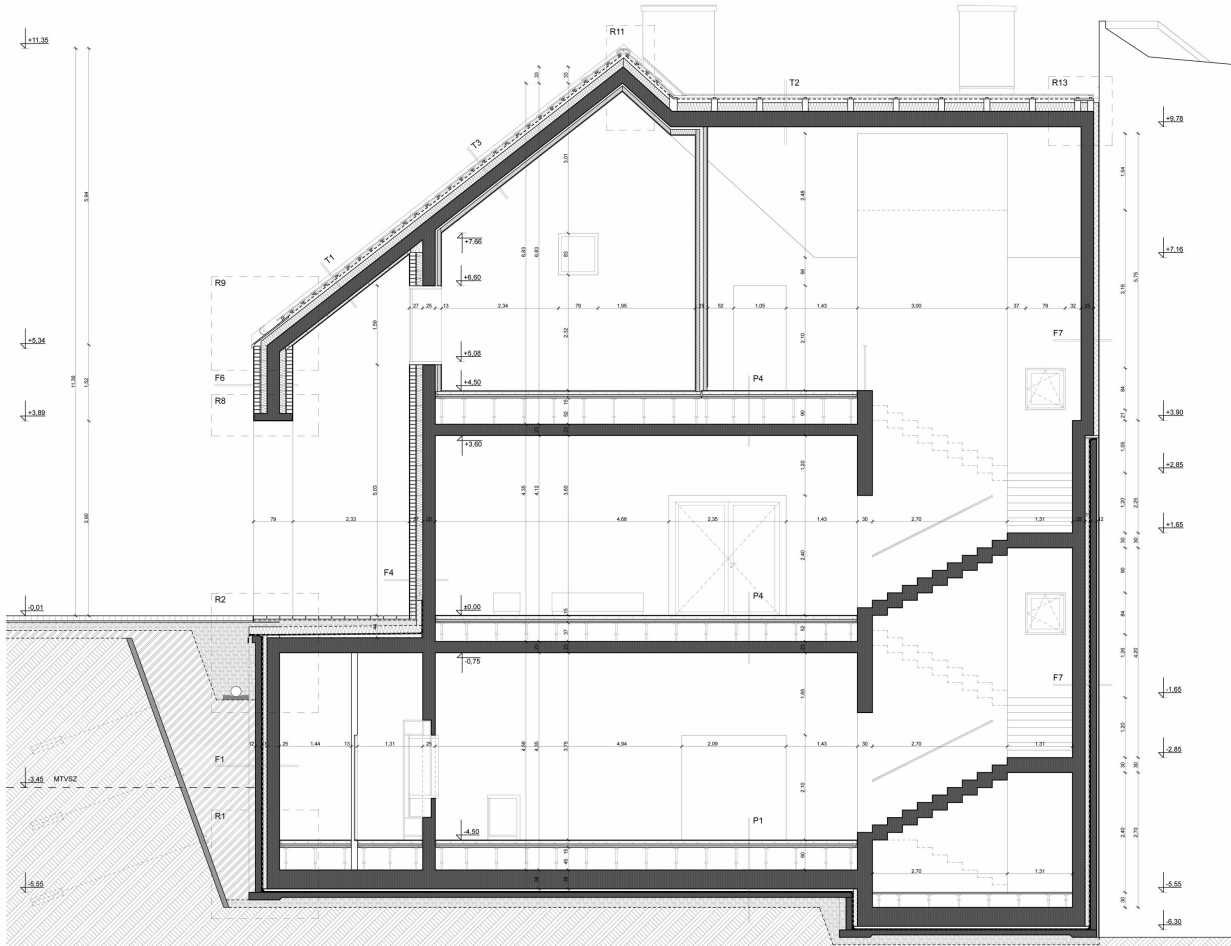
METSZET 8-8 M=1:50 ES CSOMÓPONTOK M=1:10
