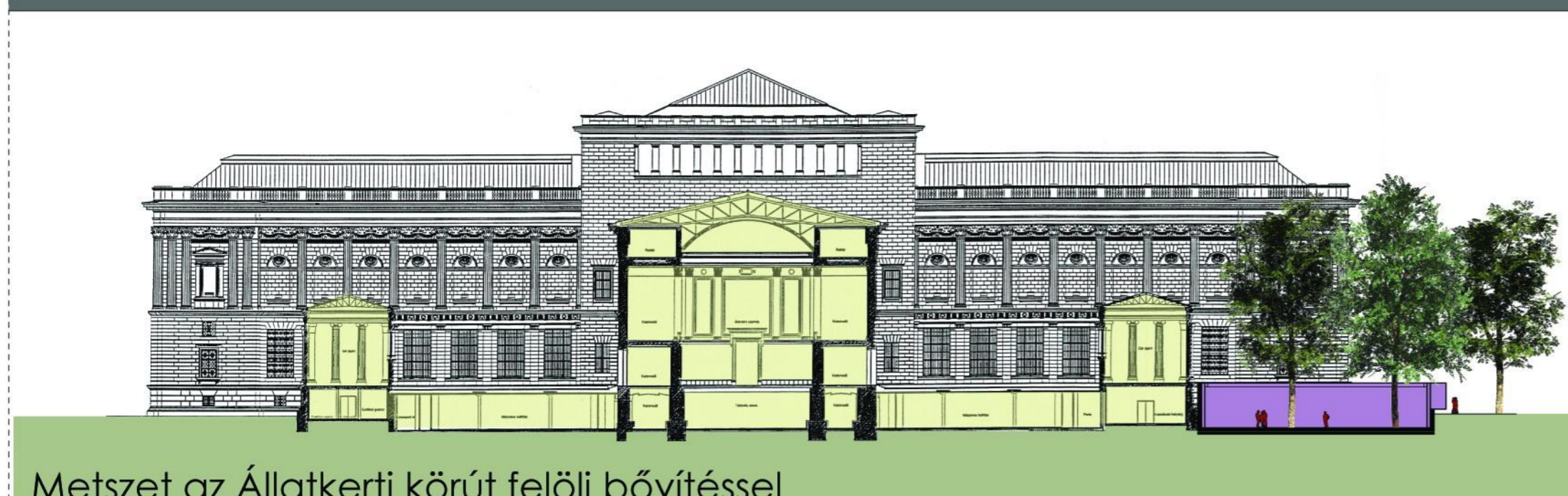
Metszet az Állatkerti körút felőli bővítéssel
