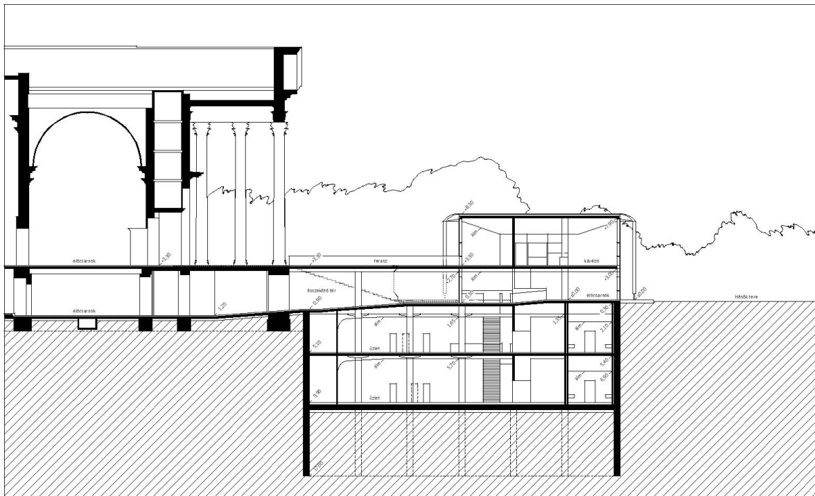
aa metszet m=1:200
