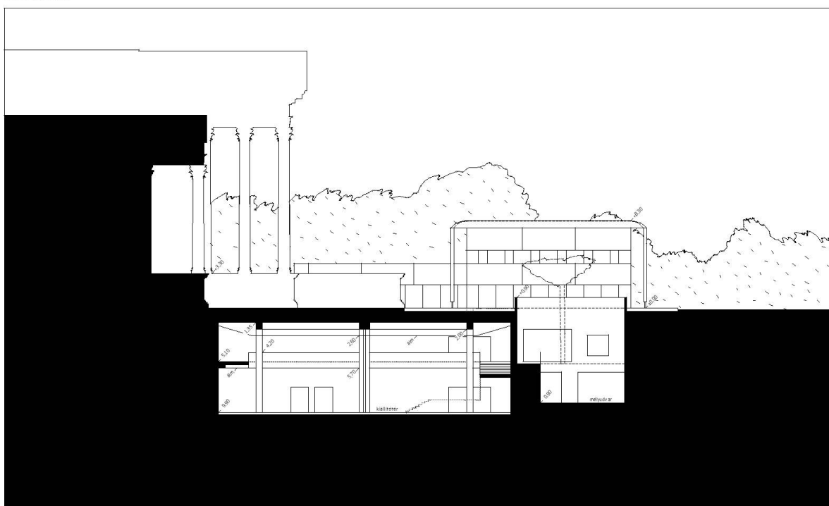
cc metszet m=1:200
