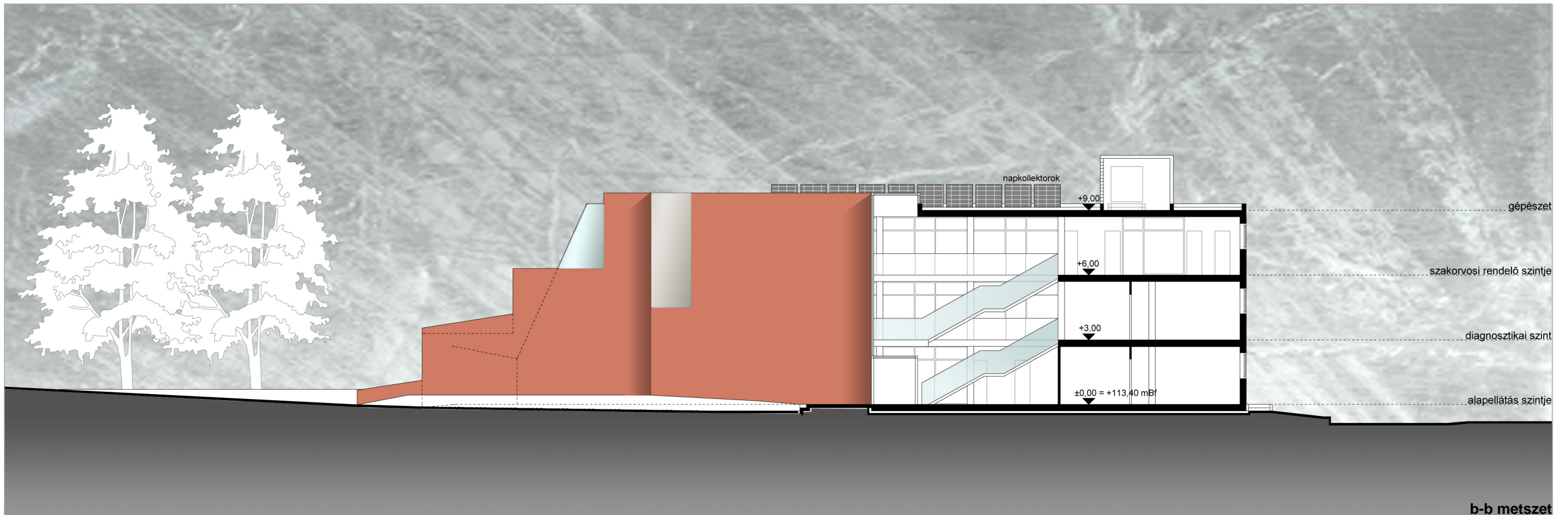
b-b metszet
