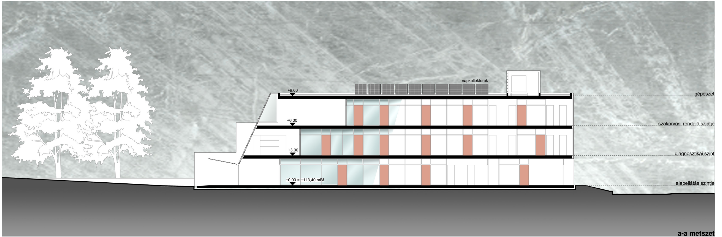
a-a metszet
