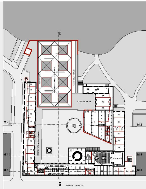
EMELETI ALAPRAJZ M1:500
