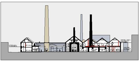
M4 METSZET M1:500
