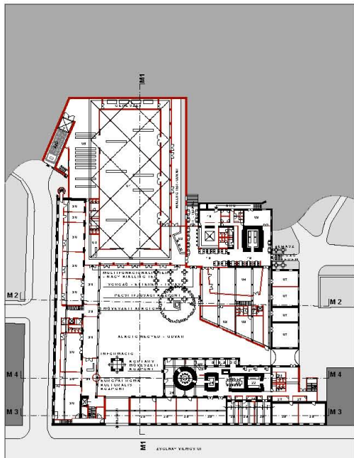
FÖLDSZINTI ALAPRAJZ M1:500
