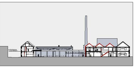
M2 METSZET M1:500
