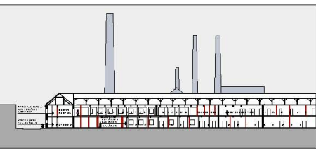
M3 METSZET M1:500
