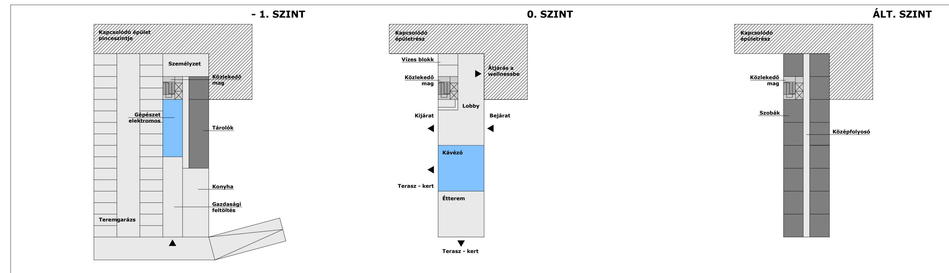
GYÓGYSZÁLLÓ FUNKCIÓ SÉMA M 1:500
