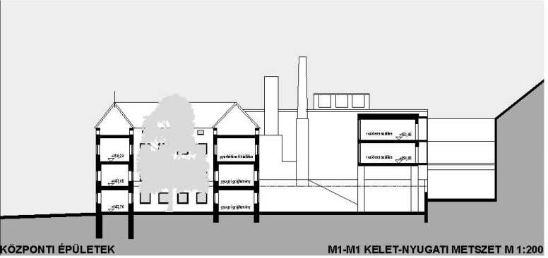
KÖZPONTI ÉPÜLETEK M1-M1 KELET-NYUGATI METSZET M 1:200
