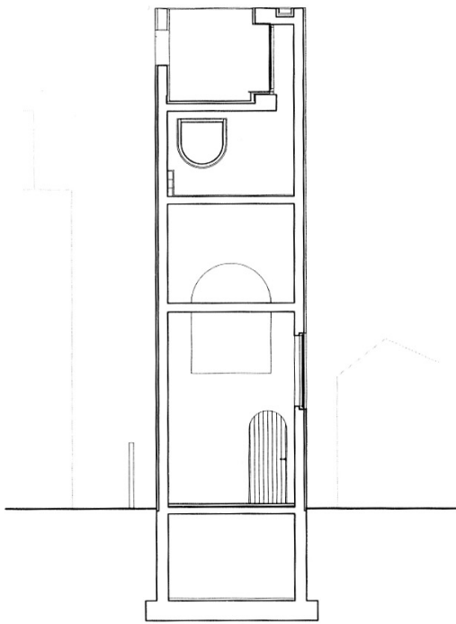
短手断面图 SECTION
