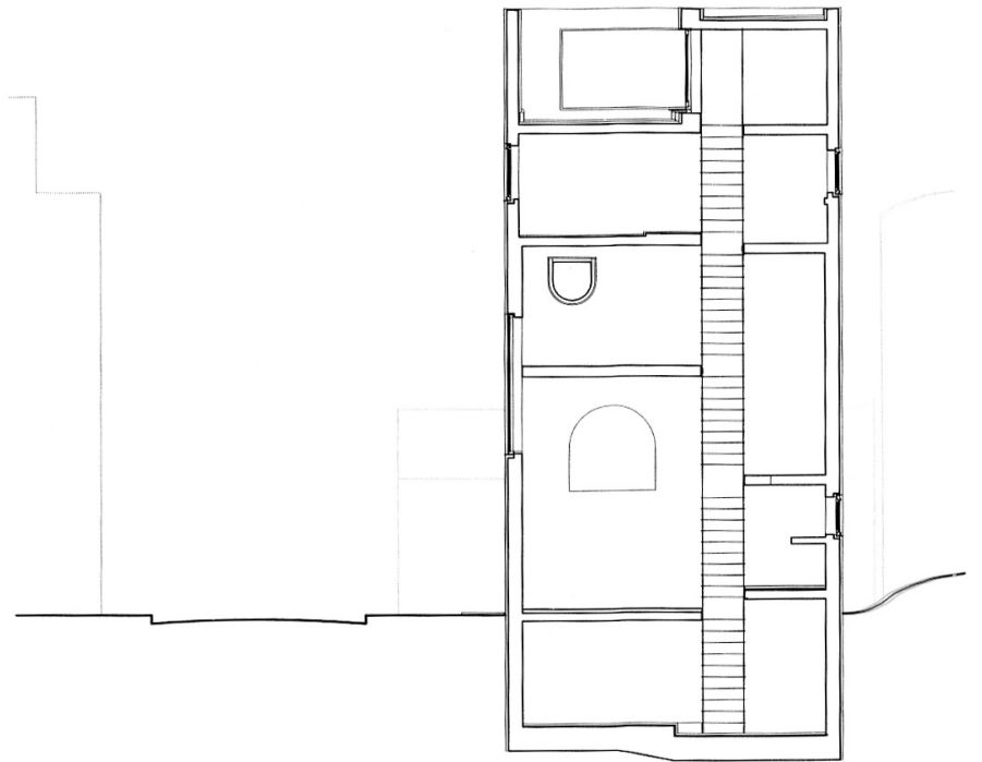
長手断面图 SECTION
