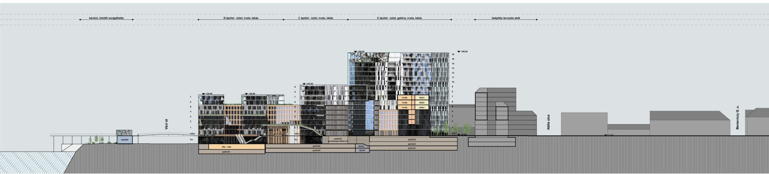
A - A METSZET LISZT FERENC UTCÁVAL PÁRHUZAMOSAN
