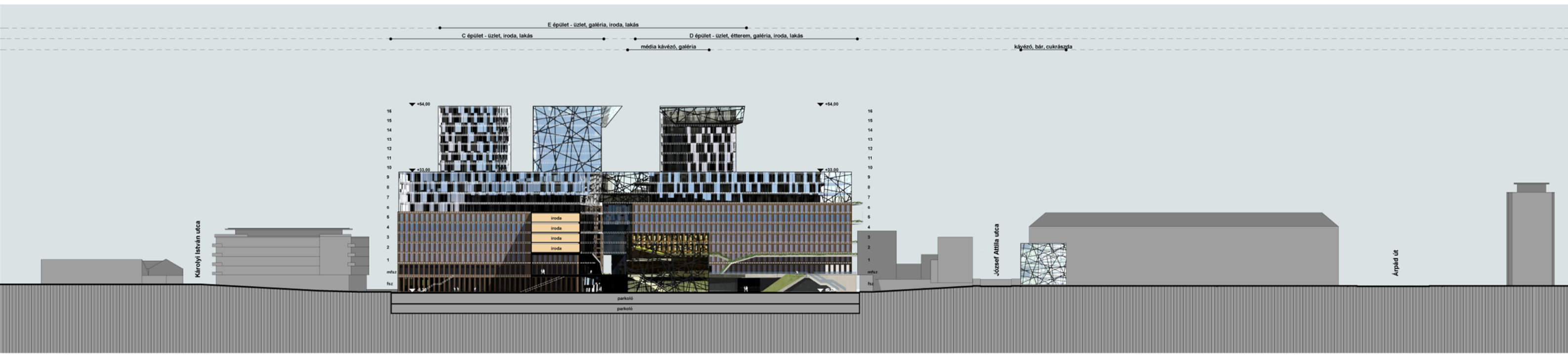
B - B METSZET VÁCI ÚTTAL PÁRHUZAMOSAN
