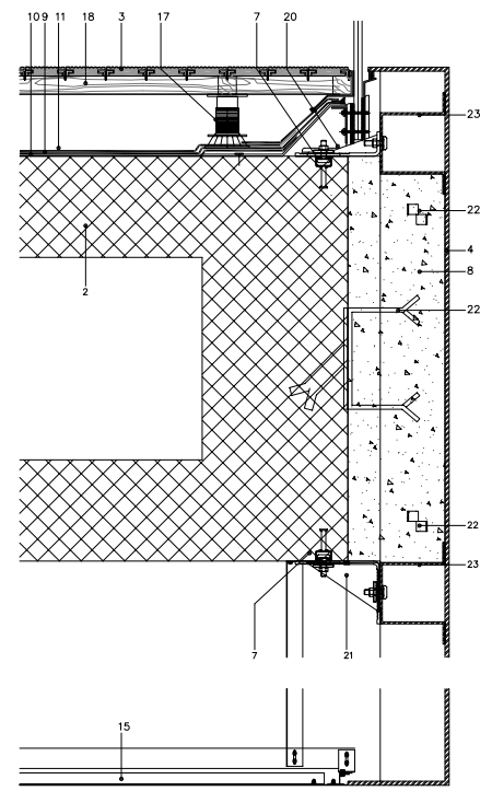
01Detalle e 1/5
