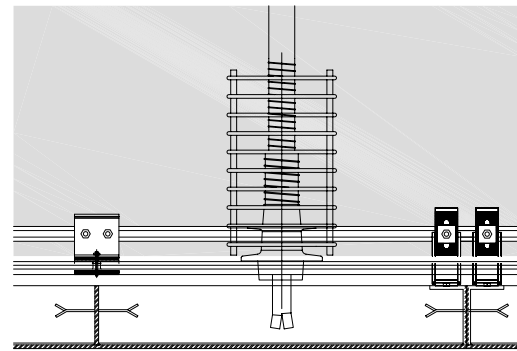
01Detalle e 1/5
