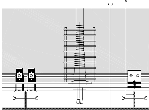
Planta e 1/5
