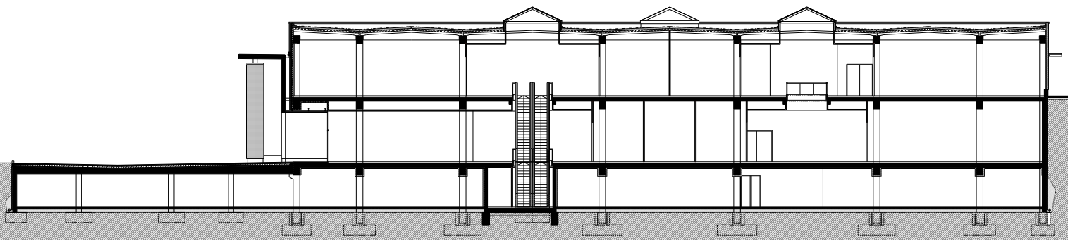
KERESZTMETSZET
