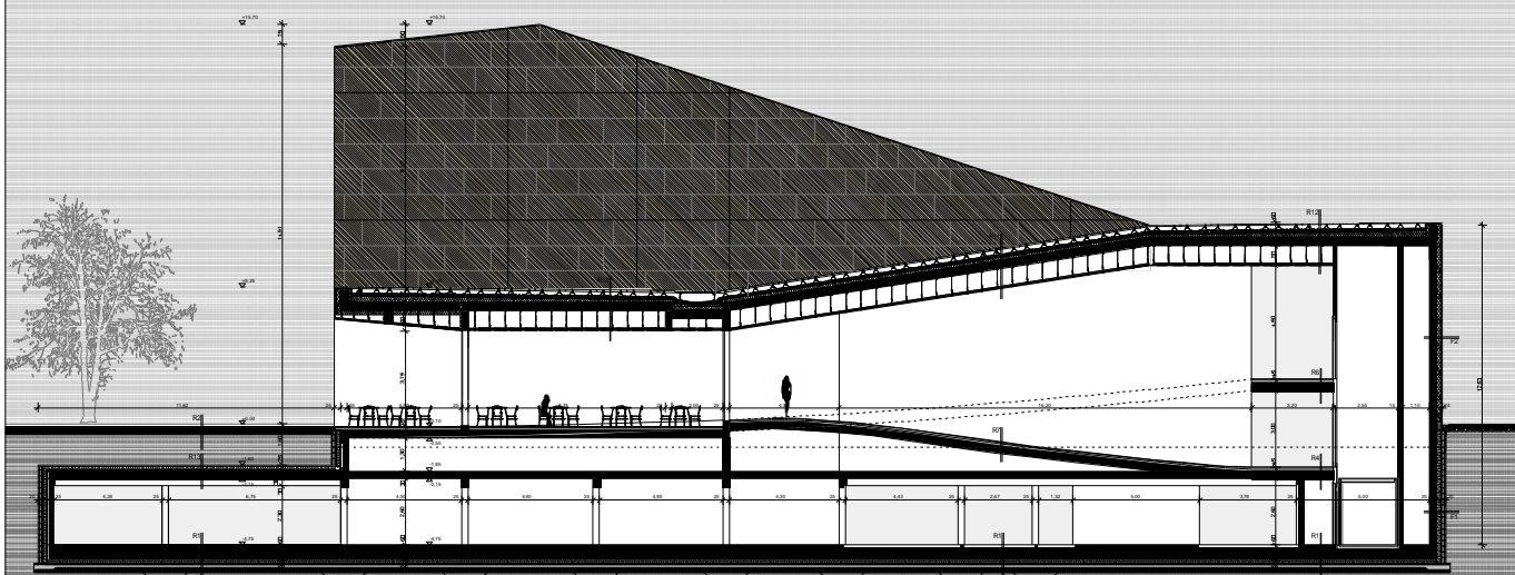
A/1 metszet
