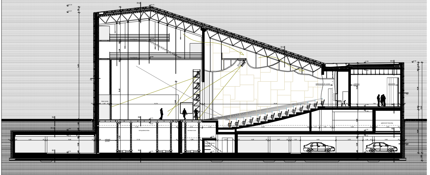
A/3 metszet
