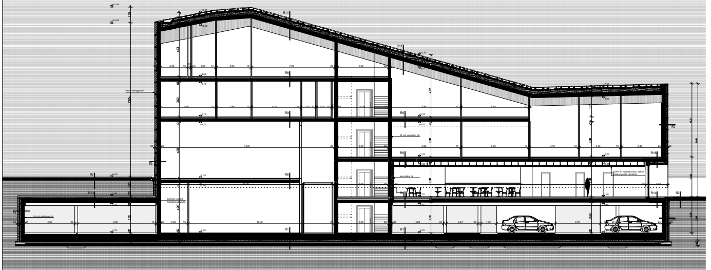
A/4 metszet
