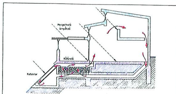
Kőtárolós napház Új-Mexikóban (17)
