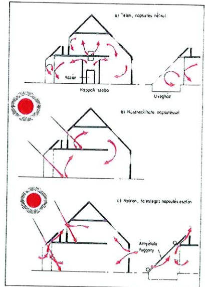
Szentendrei szolárház (az "Év lakóháza" díjas) (1985) tervező: Dr. Kuba Gellért építészmérnök (17)
