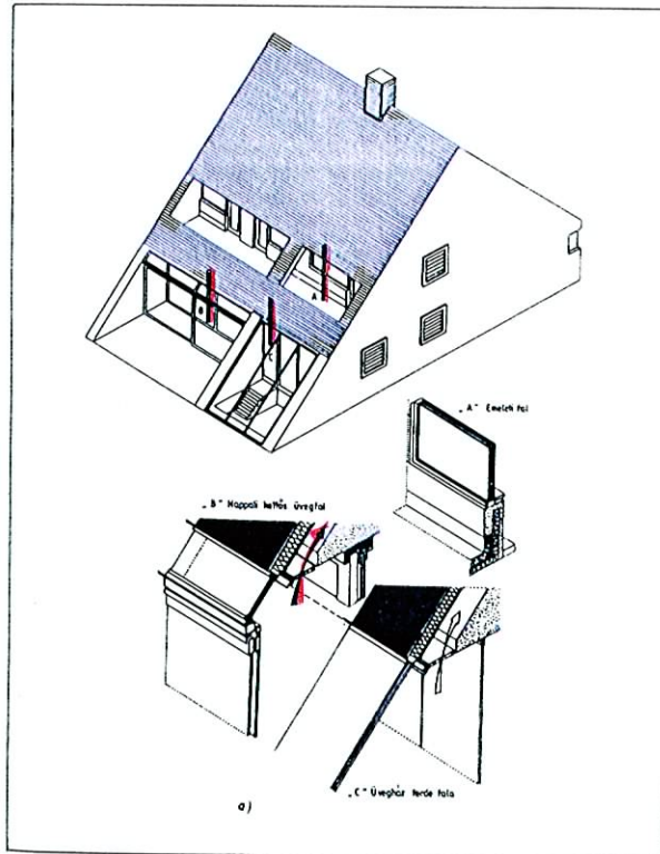
Üvegezett előtérrel épült ház
