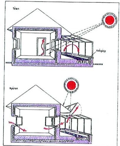
Télikert hőhasznosítása, működtetése (17)
