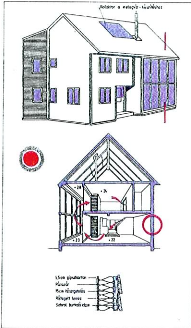
Üvegezett előtérrel épült ház
