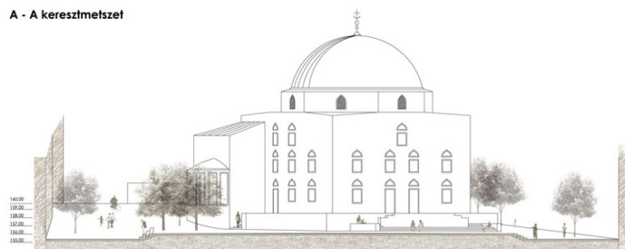
A - A keresztmetszet
